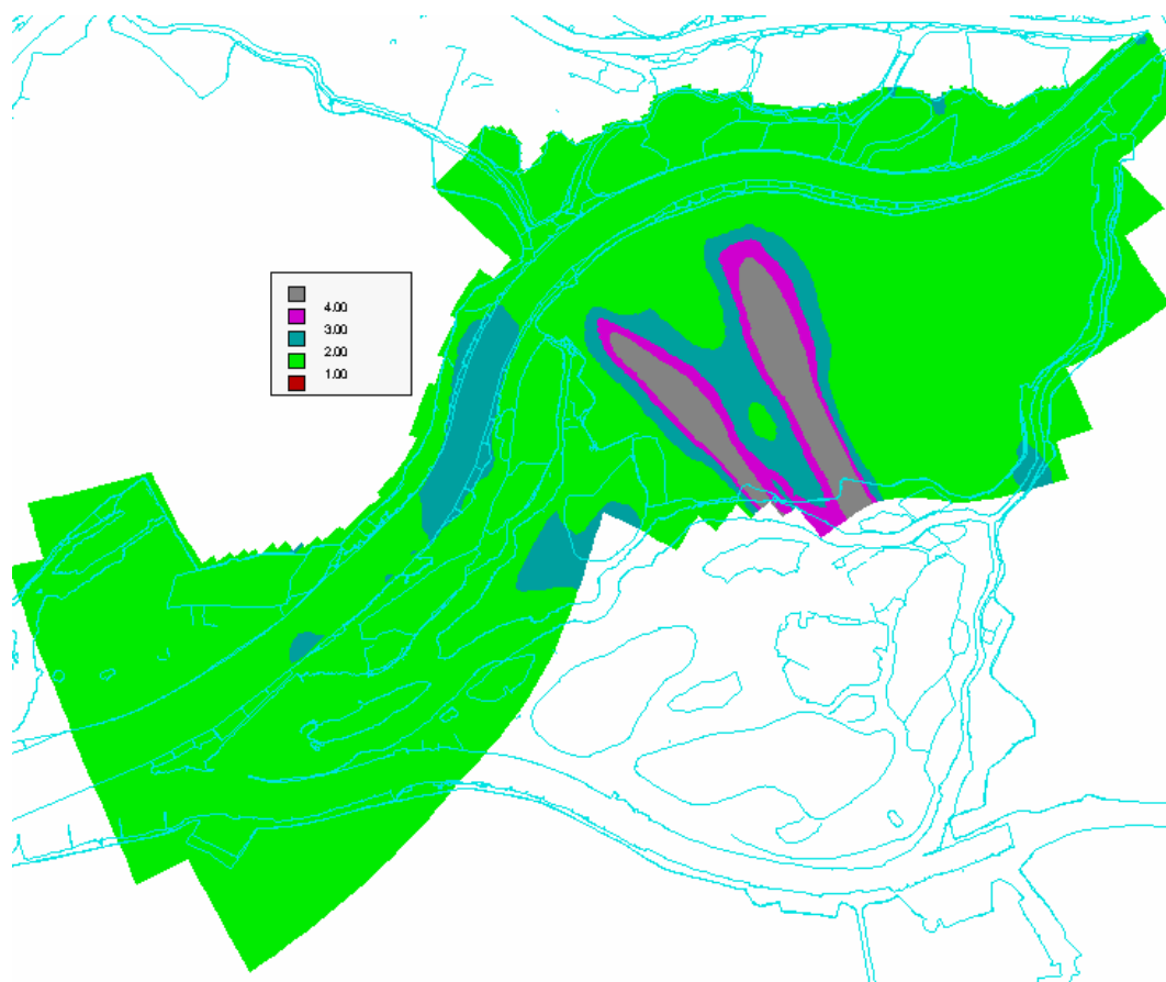
Figuur 3.16. Lengte-breedteverhoudingen van roostercellen voor de Nieuwe Merwede.
