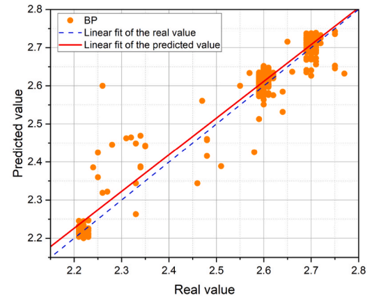
b) BP
