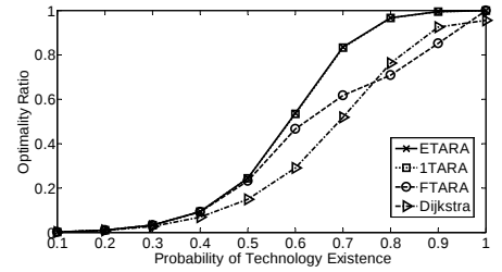
(d) GÉANT
