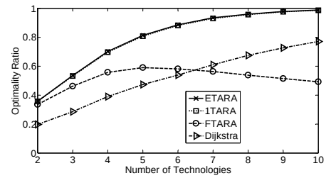
(d) GÉANT
