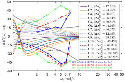
(d) Phase, \Delta\sigma_u^2
