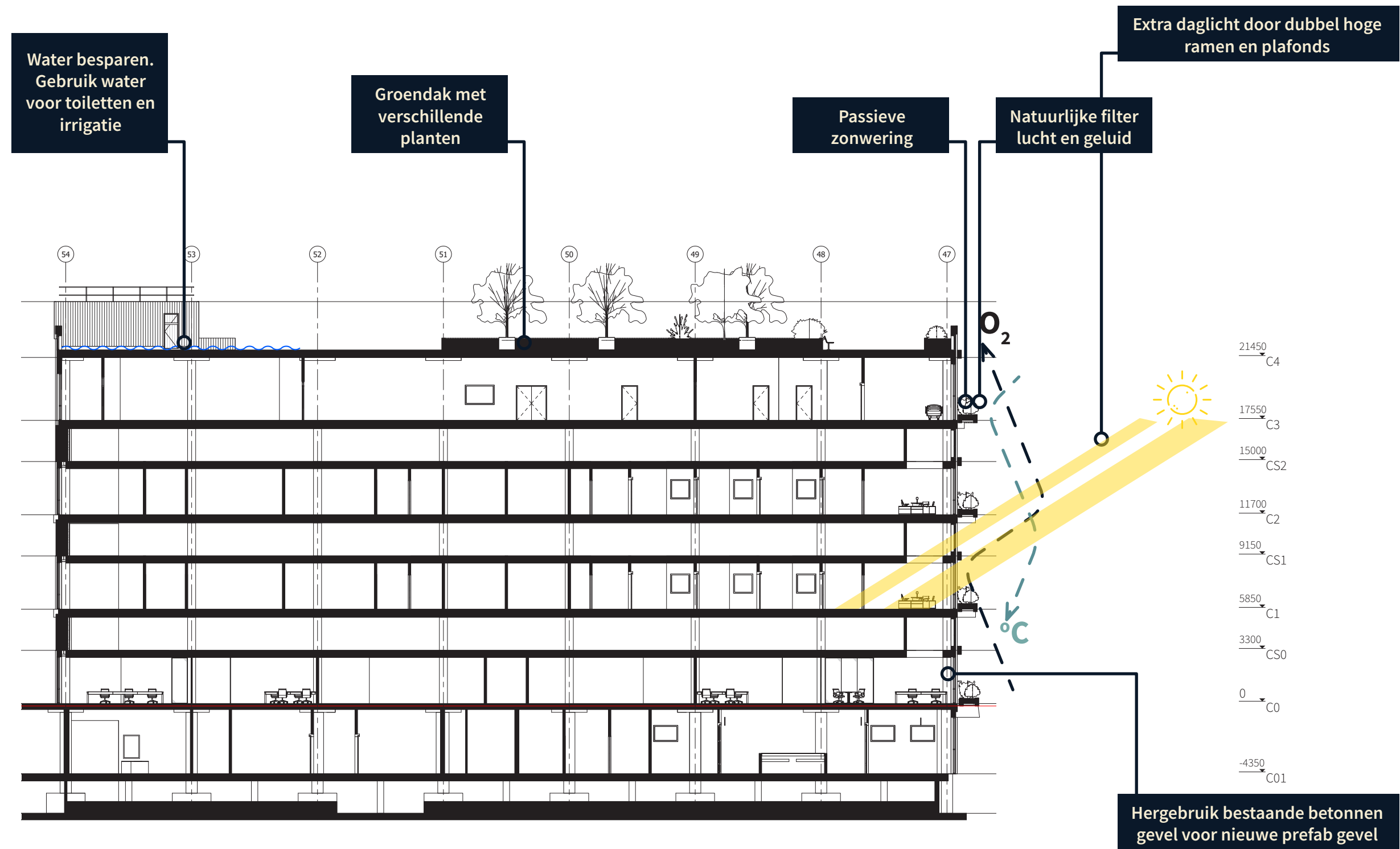
DOORSNEDE BB'
