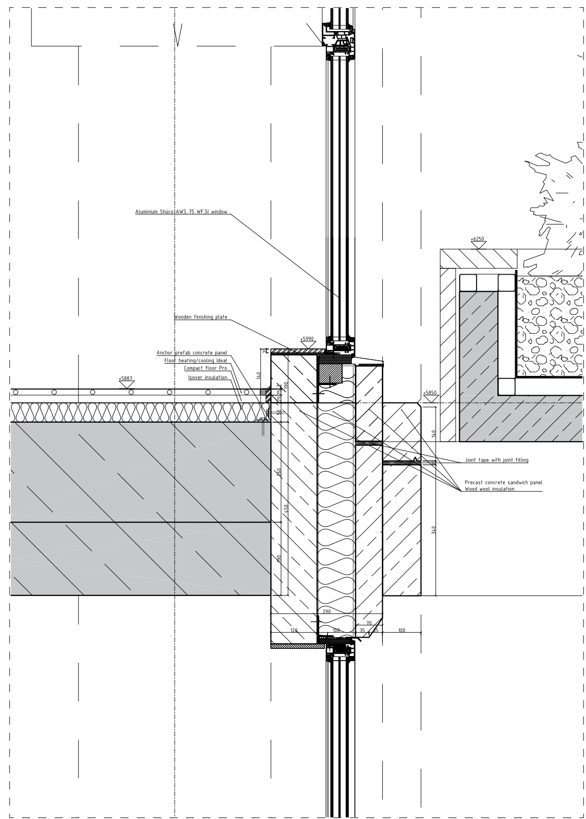
DETAIL KANTOOR VLOER
