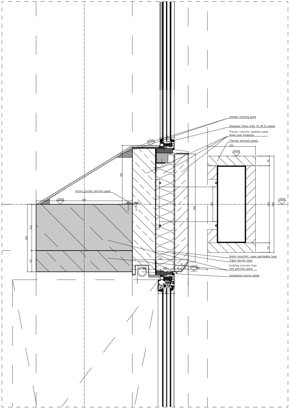
DETAIL SERVICE VLOER
