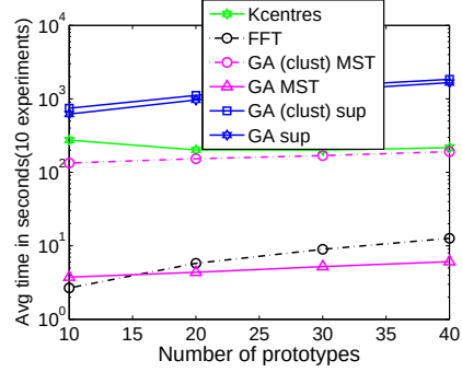
(d) MNIST
