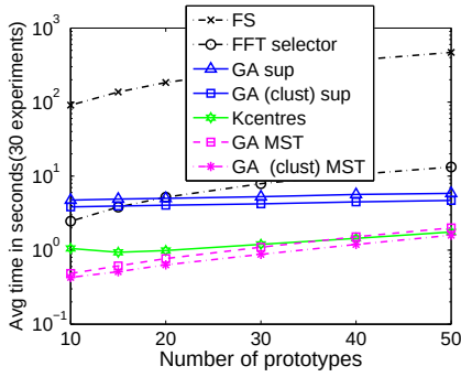
(a) Zongker
