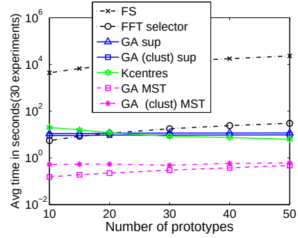
(b) Pendigits
