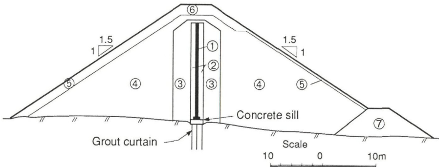
Fig. 3.7 Vestredalstjern Dam
