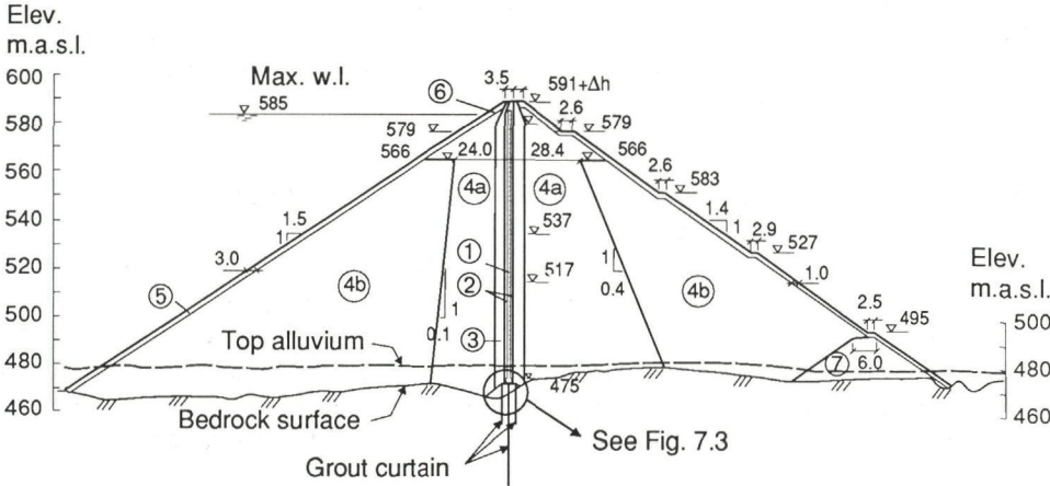
Fig. 7.2 Storglomvatn Dam
