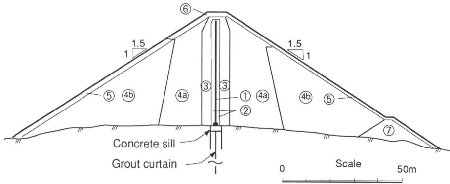
Fig. 3.4 Styggevatn Dam
