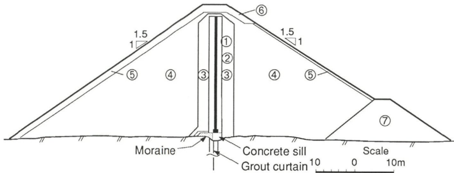
Fig. 3.6 Katlavatn Dam
