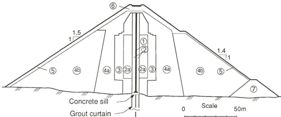
Fig. 3.5 Riskallvatn Dam
