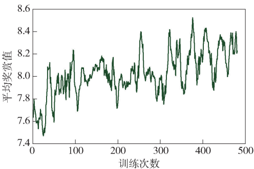
图 9 平均奖赏值变化图
