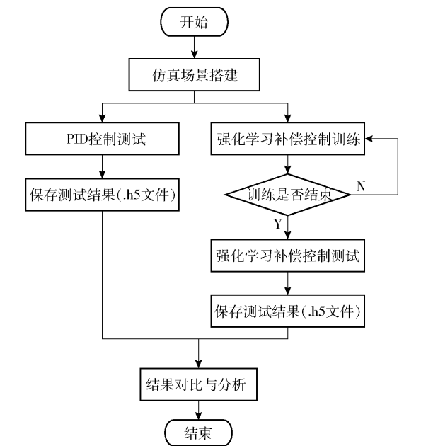
图 7 仿真实验流程图
