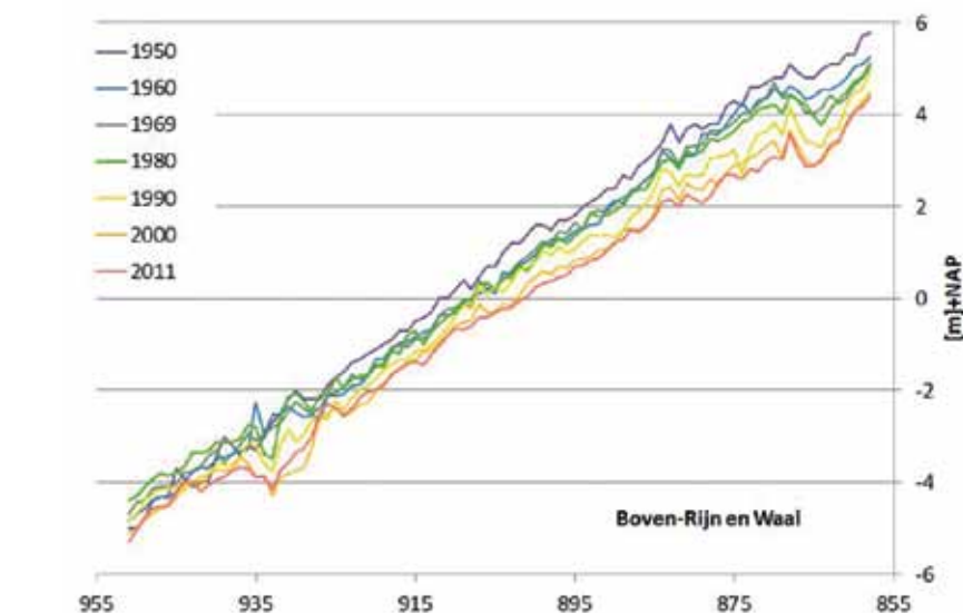
Figuur 3 De ontwikkeling van het zomerbed sedert 1950 (op basis van gegevens van Arjen Sieben, Rijkswaterstaat): voortschrijdende insnijding en kanteling van het rivierlangsprofiel in respons op interventies in het stroomgebied en de normalisaties.
