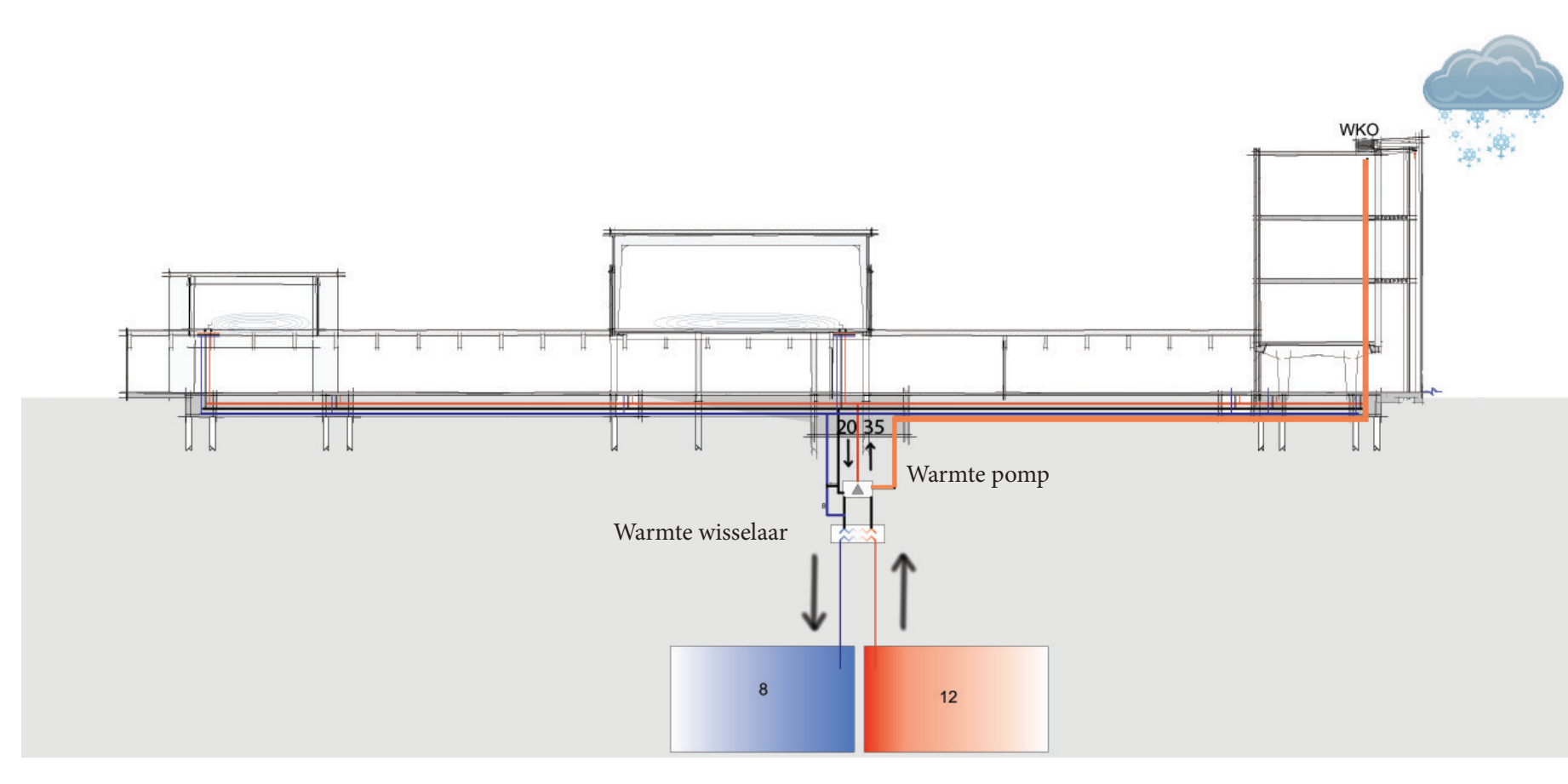
Verwarmings- & koelingsprincipe
