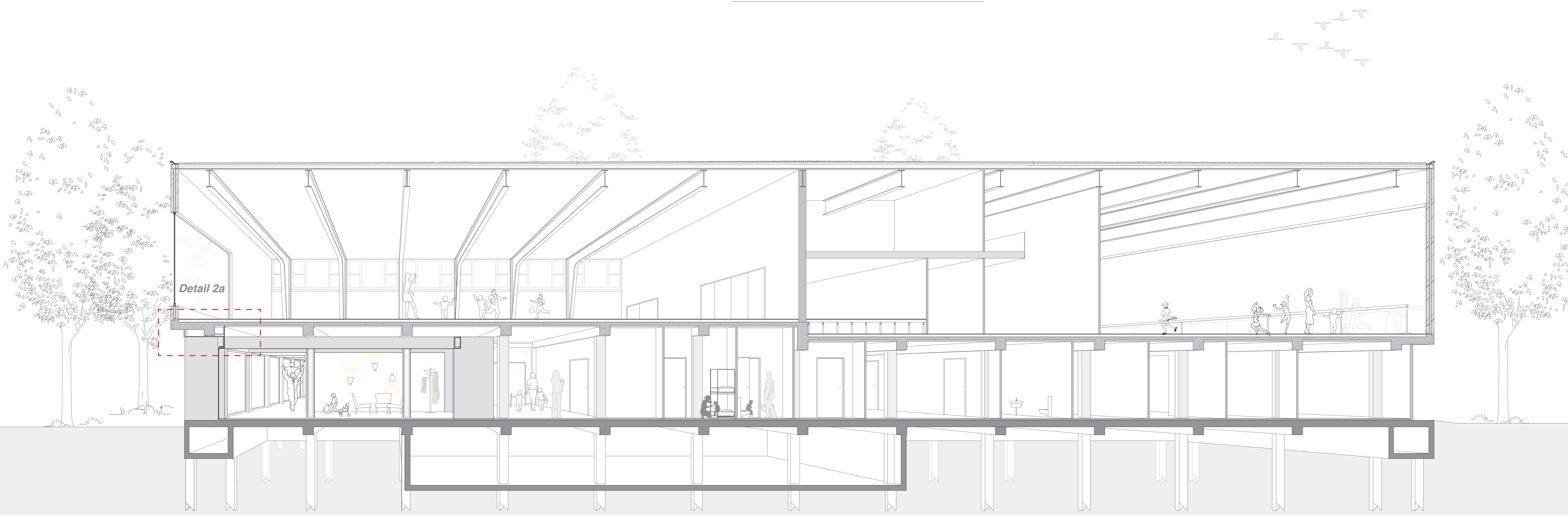
Doorsnede Midden 1:100
