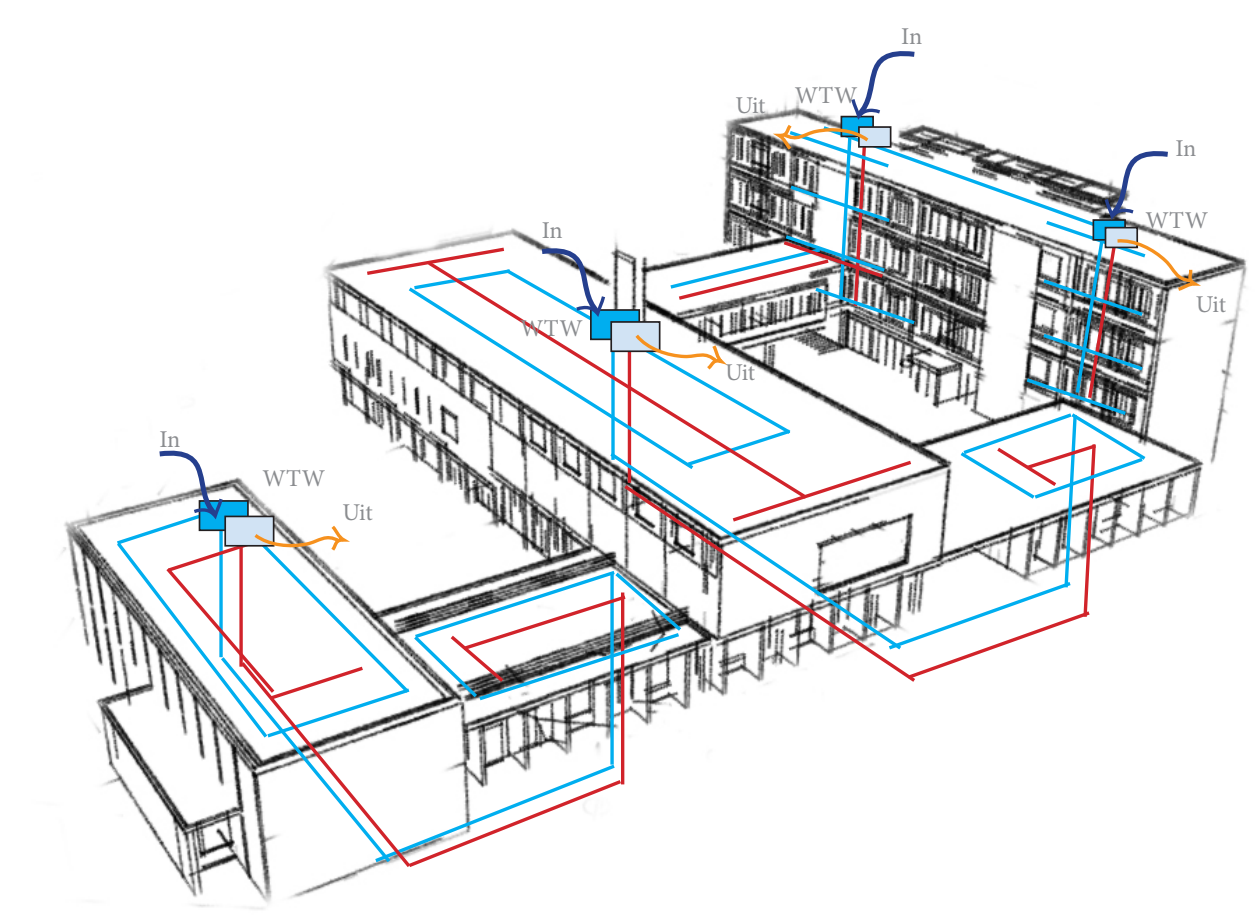
Ventilatieprincipe
