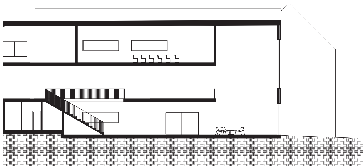
DOORSNEDE CC'
