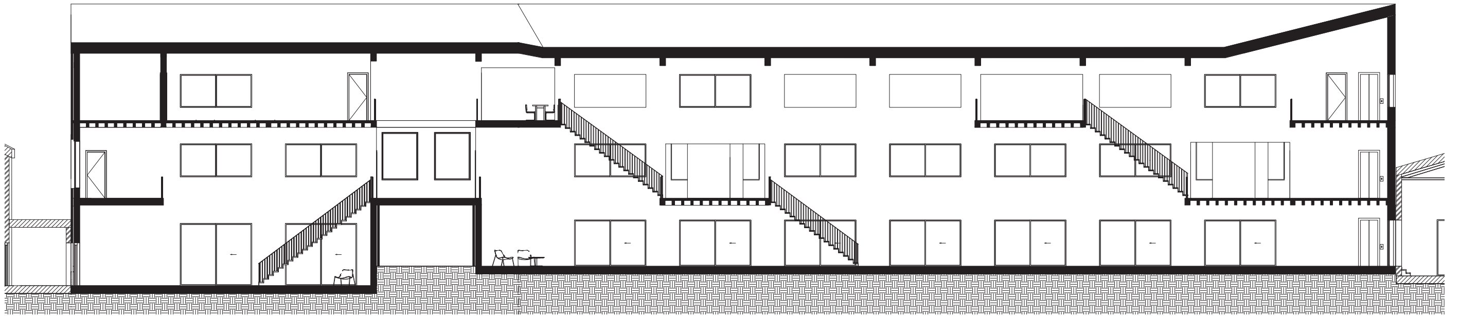
DOORSNEDE AA'
