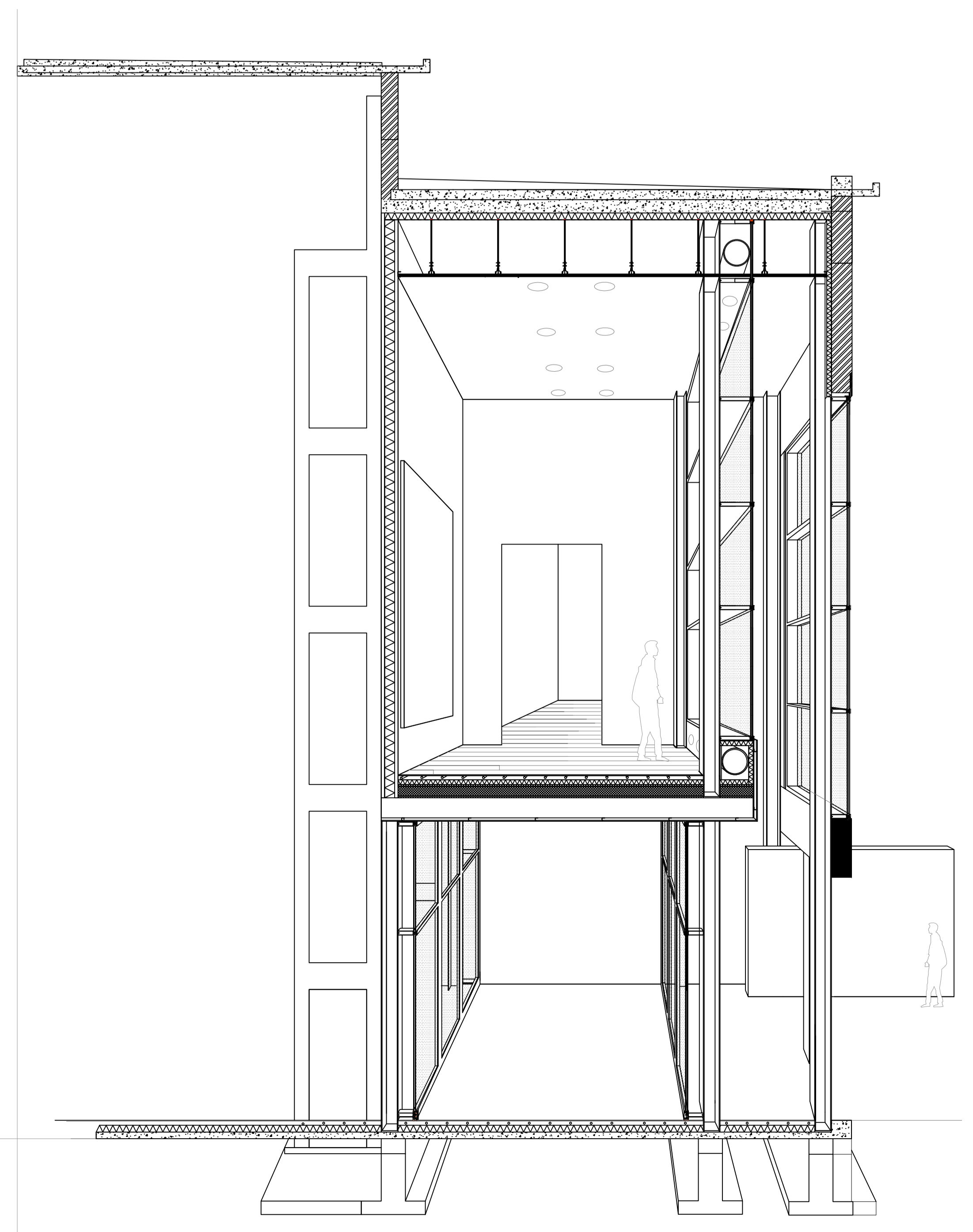
doorsnede entree _ 1:50
