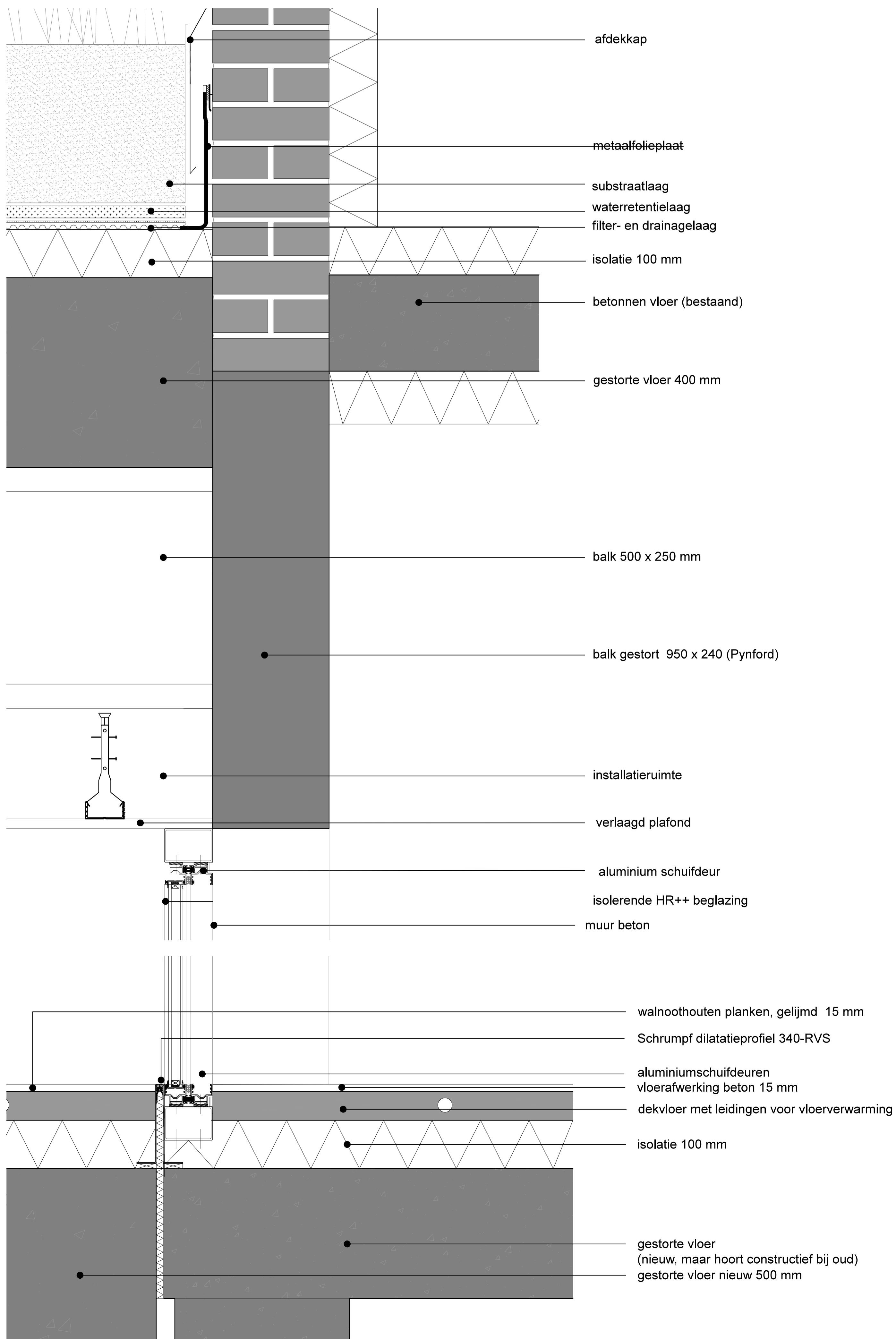
detail 5 en 6. _ 1:5
