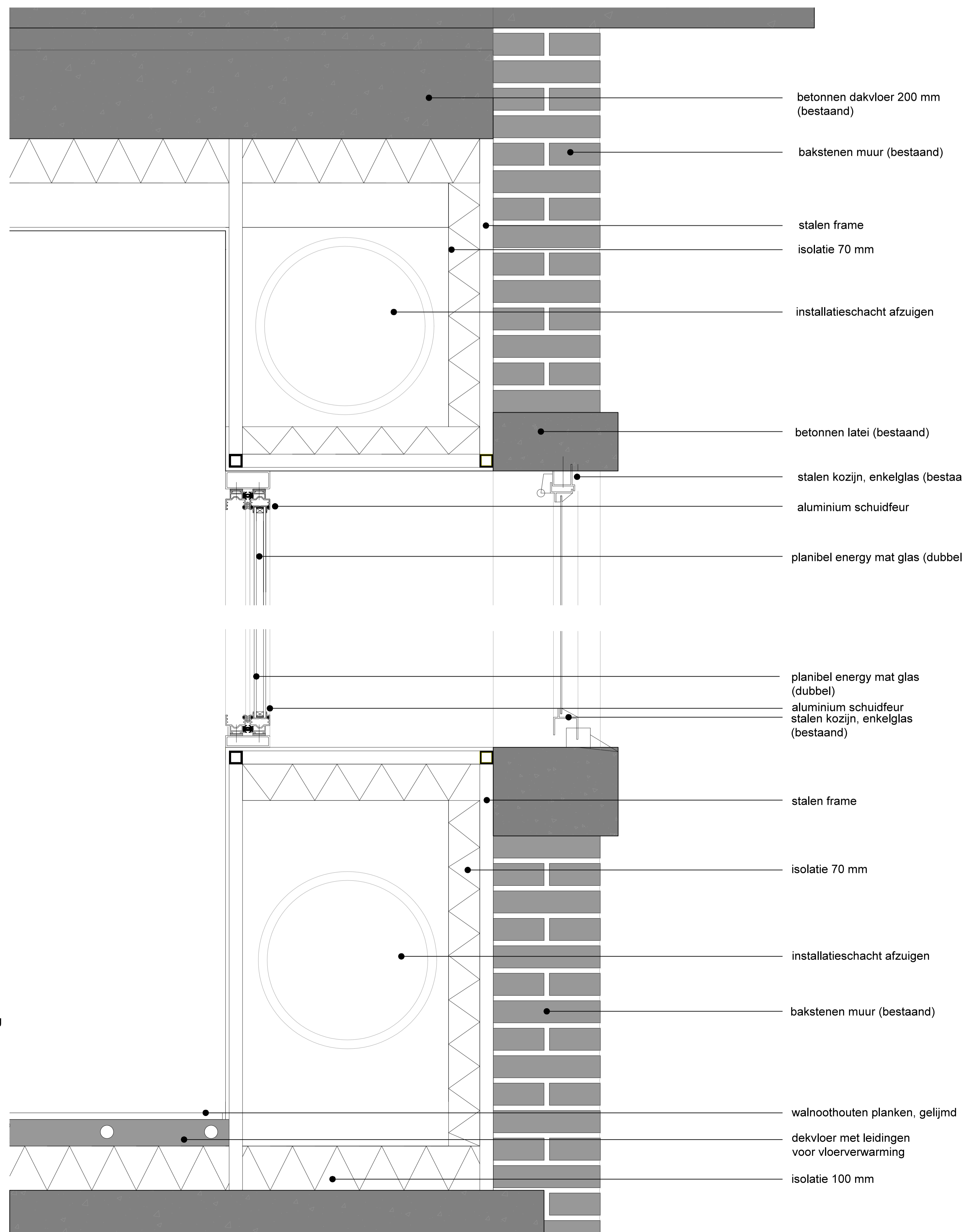
detail 7 en 8. _ 1:5
