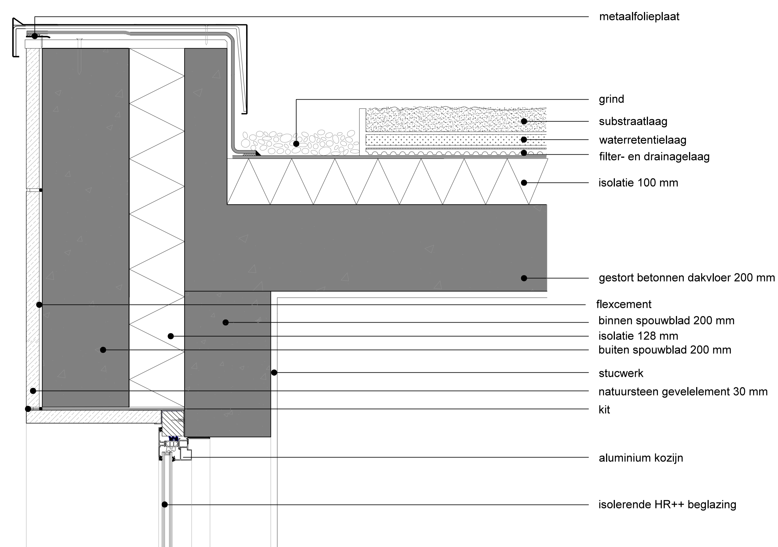
detail 1 en 2. _ 1:5
