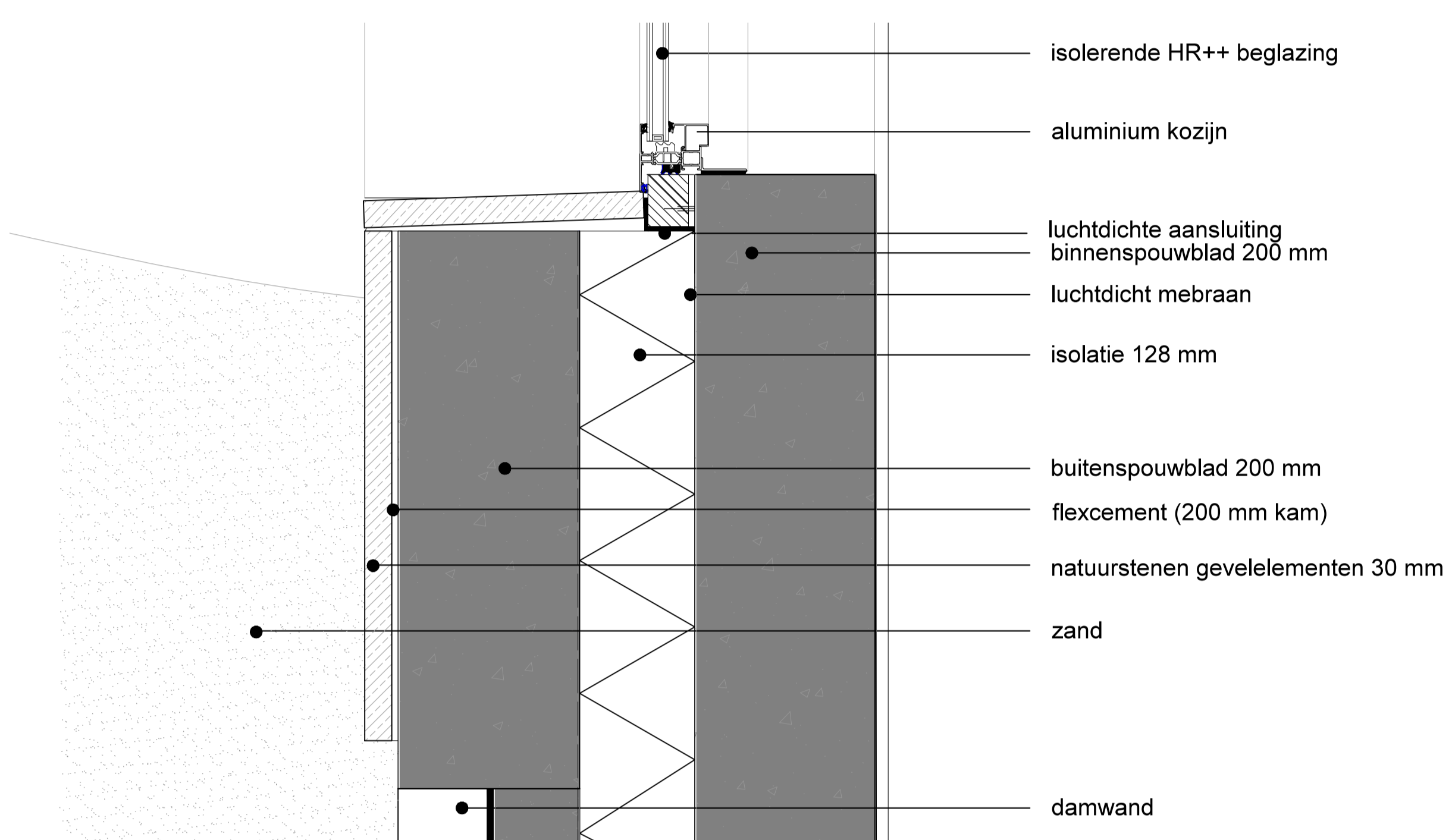
detail 5 en 6. _ 1:5
