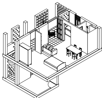
maisonette living upstairs 57 m 2
