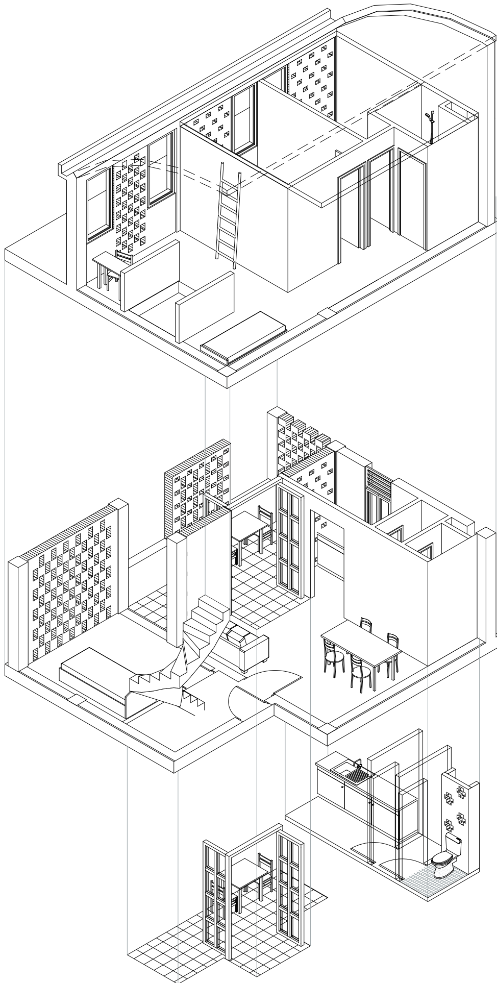
PENTHOUSE I AXONOMETRY // 1:100
