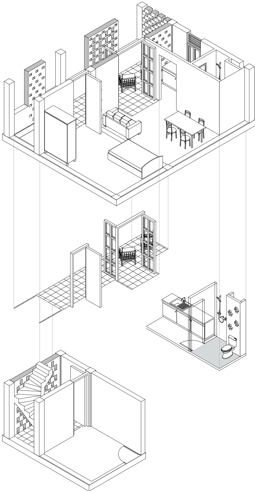
MAISONETTE LIVING UPSTAIRS AXONOMETRY // 1:100
