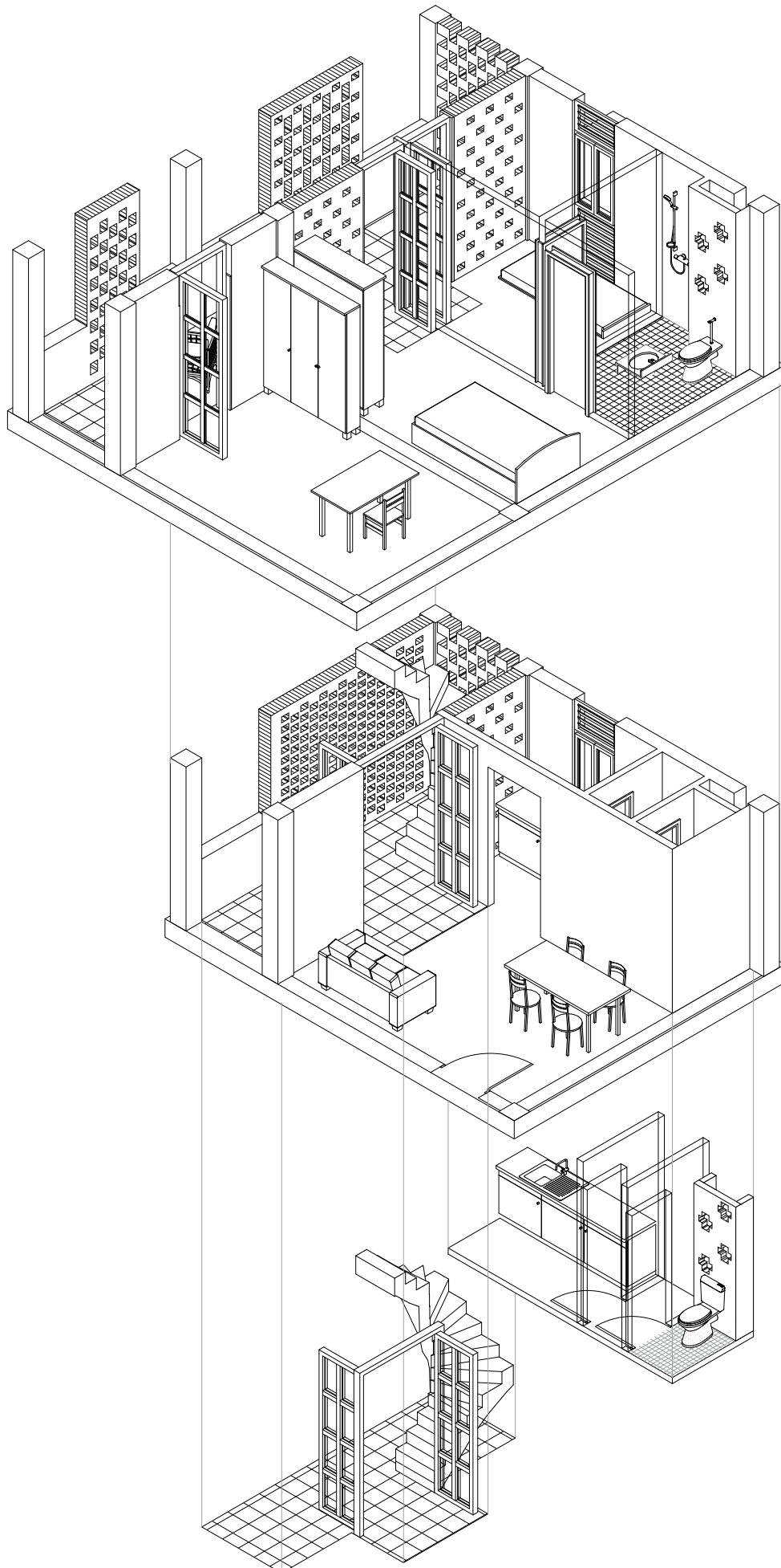
MAISONETTE UNIT AXONOMETRY // 1:100
