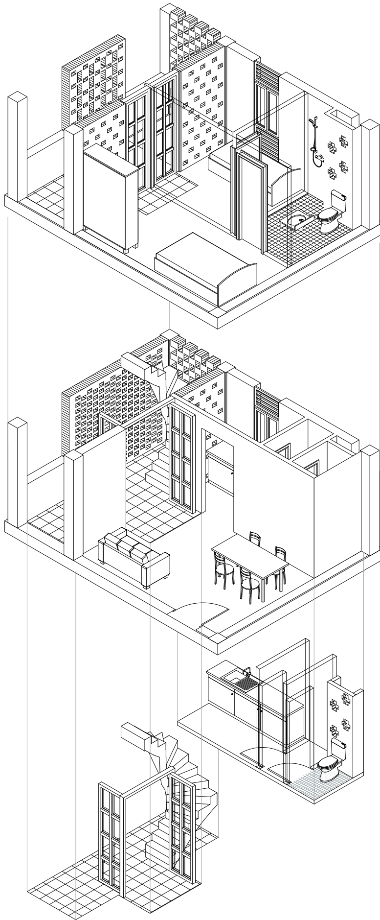
MAISONETTE UNIT AXONOMETRY // 1:100
