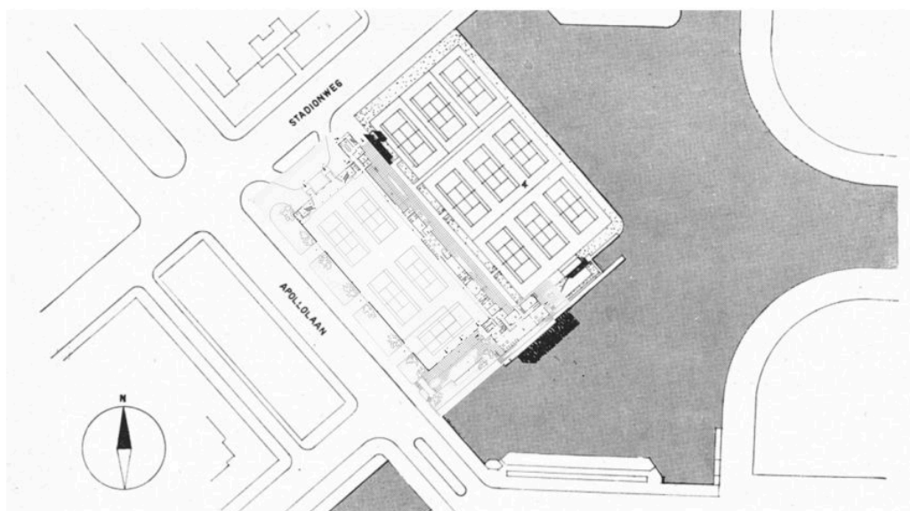
Afbeelding 10.1.10A Apollohal in Amsterdam, ontwerp Albert Boeken, 1934, boven: luchtfoto, 1957 (Foto Aviodrome, Lelystad), en ontwerp van het terrein (onder: bron).
