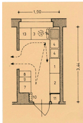
14.2 Plattegrond van de Frankfurter Küche uit Küche Frankfurter Küche – Ullis Culinaria ( ulis-culinaria.de ); niet beschikbaar voor vrij hergebruik
