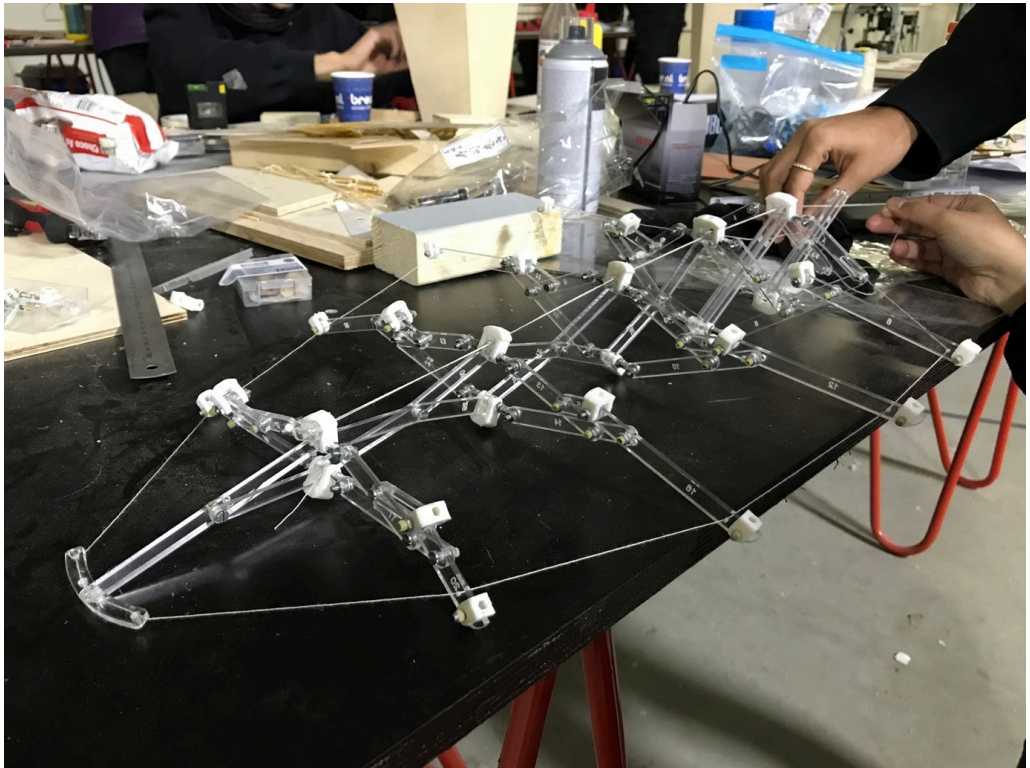
Fig.5 functiemodel van een zonnenuif 1:5 (door Kritika Agarwal, Priyadarshini Nanda, Shweta Kamble, Pierre Kauter en Okan Türkan, gebruik met toestemming).
