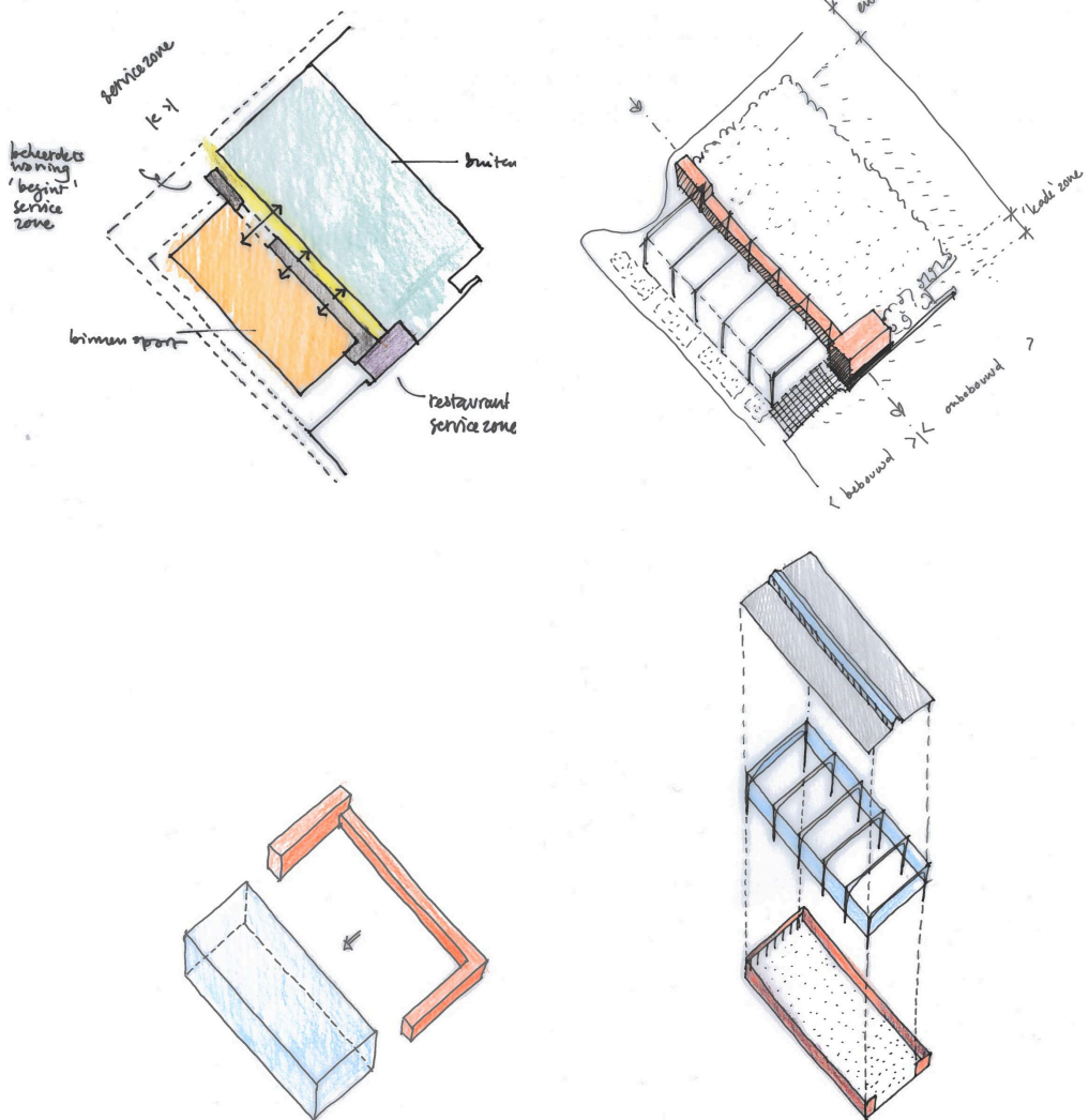
Afbeelding 10.1.10B Architectonische plananalyse van de Apollohal door Esther Gramsbergen, 2019, analysestap 'interpreteren': op basis van de tekening van het terrein zijn in de analysestap 'ordening herkennen' eerst ordeningstekeningen gemaakt van de basisbegrippen 'gebruik' (linksboven) en 'ruimte' (linksonder en rechtsonder), op basis waarvan een driedimensionale verklarende tekening is gemaakt voor het basisbegrip 'compositie' van het terrein en de bouwmassa (rechtsboven), met behulp van de tekentechnieken 'reduceren', 'toevoegen' en 'construeren'.
