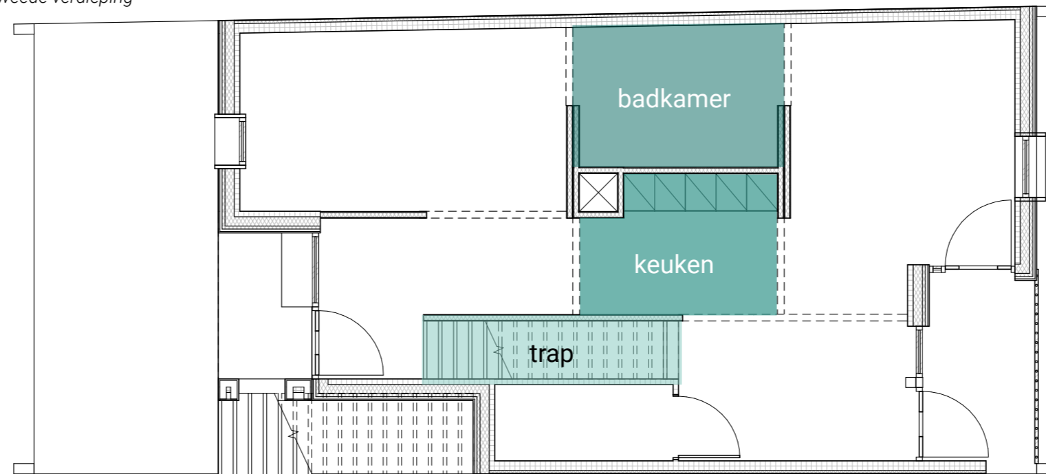
eerste verdieping
