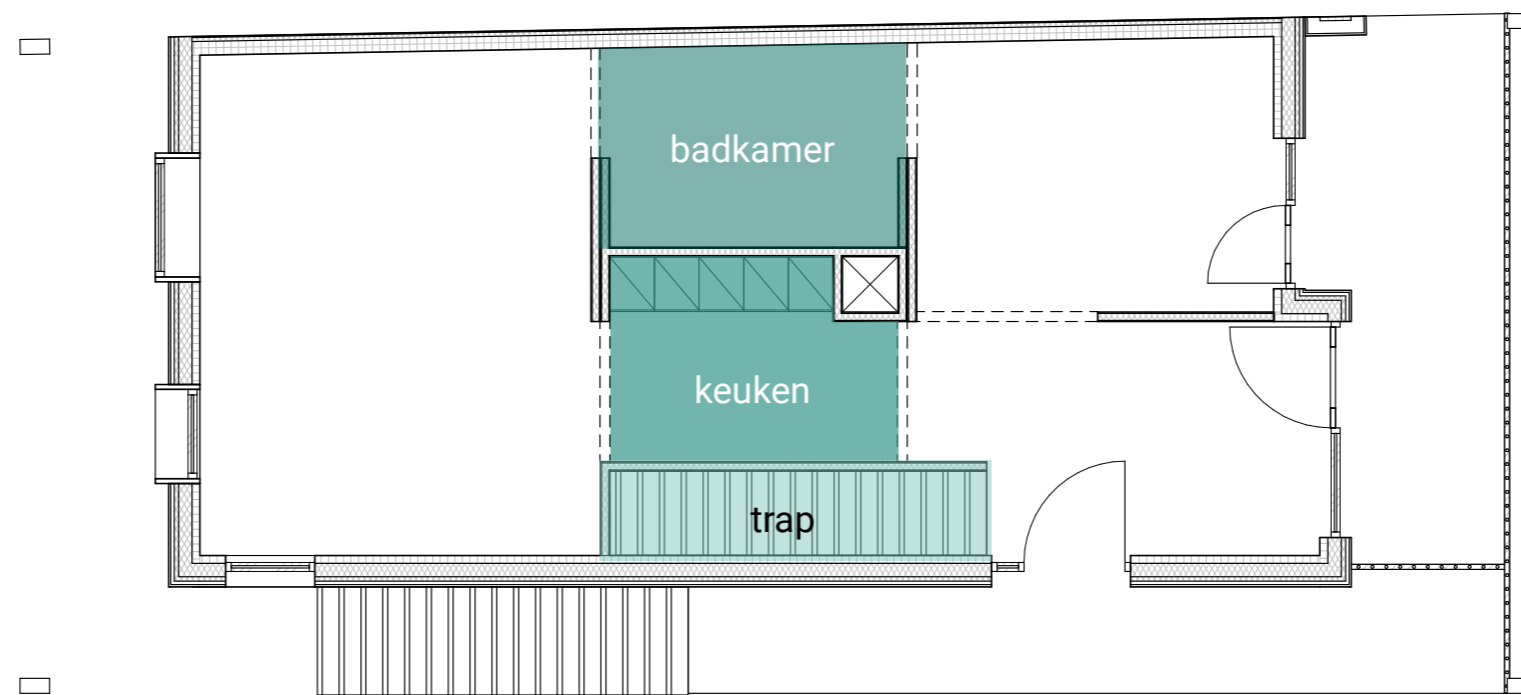
tweede verdieping
