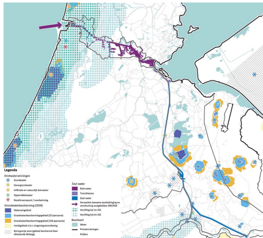
FIG. 1.4.9 Mogelijke verzilting als gevolg van een stijgende zeespiegel en bestaande gebieden voor drinkwaterwingebieden (data: Atlas van de Regio)
