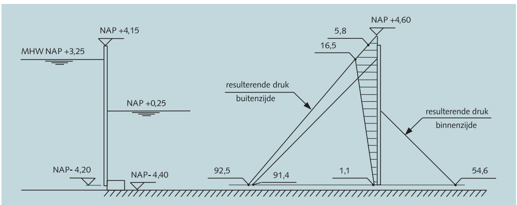
Figuur B8.2 Maatgevende waterdrücken op deuren
