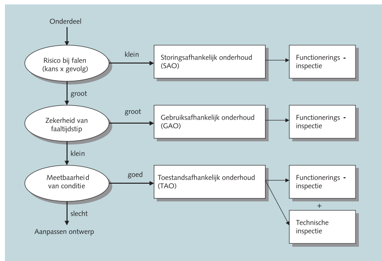
Figuur B6.6 Beslisdiagram onder- houds- en inspectiestra- tegie
