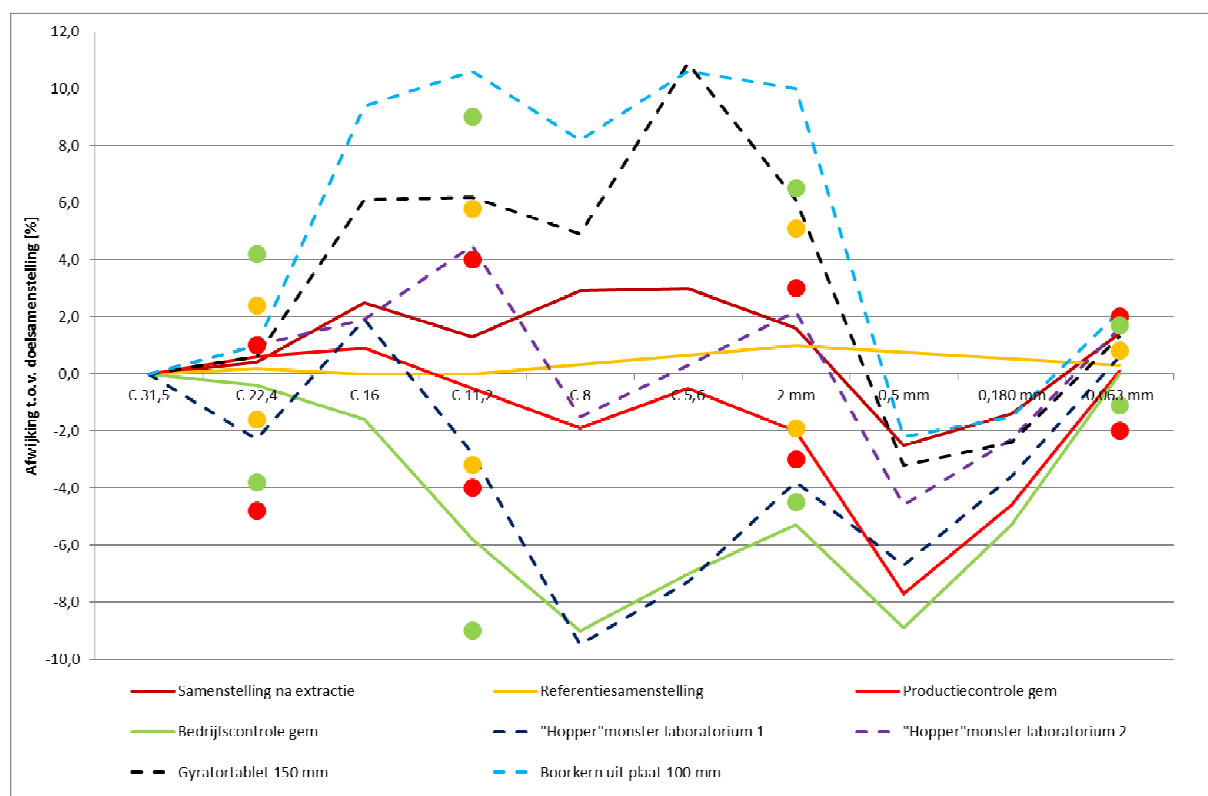
Figuur 3 Afwijking samenstelling t.o.v. doelsamenstelling
