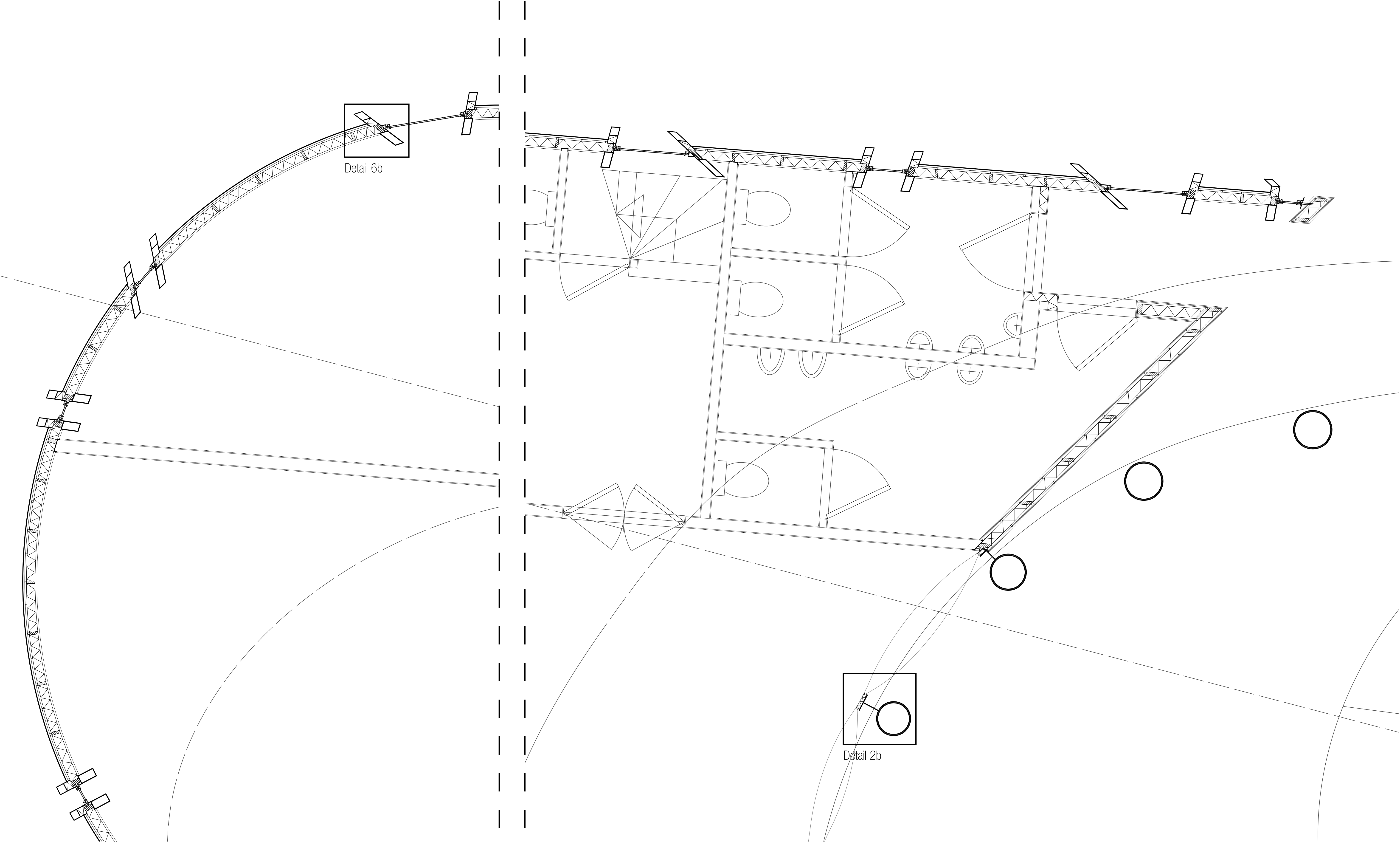
Horizontale doorsnede winkel Schaal 1:20
