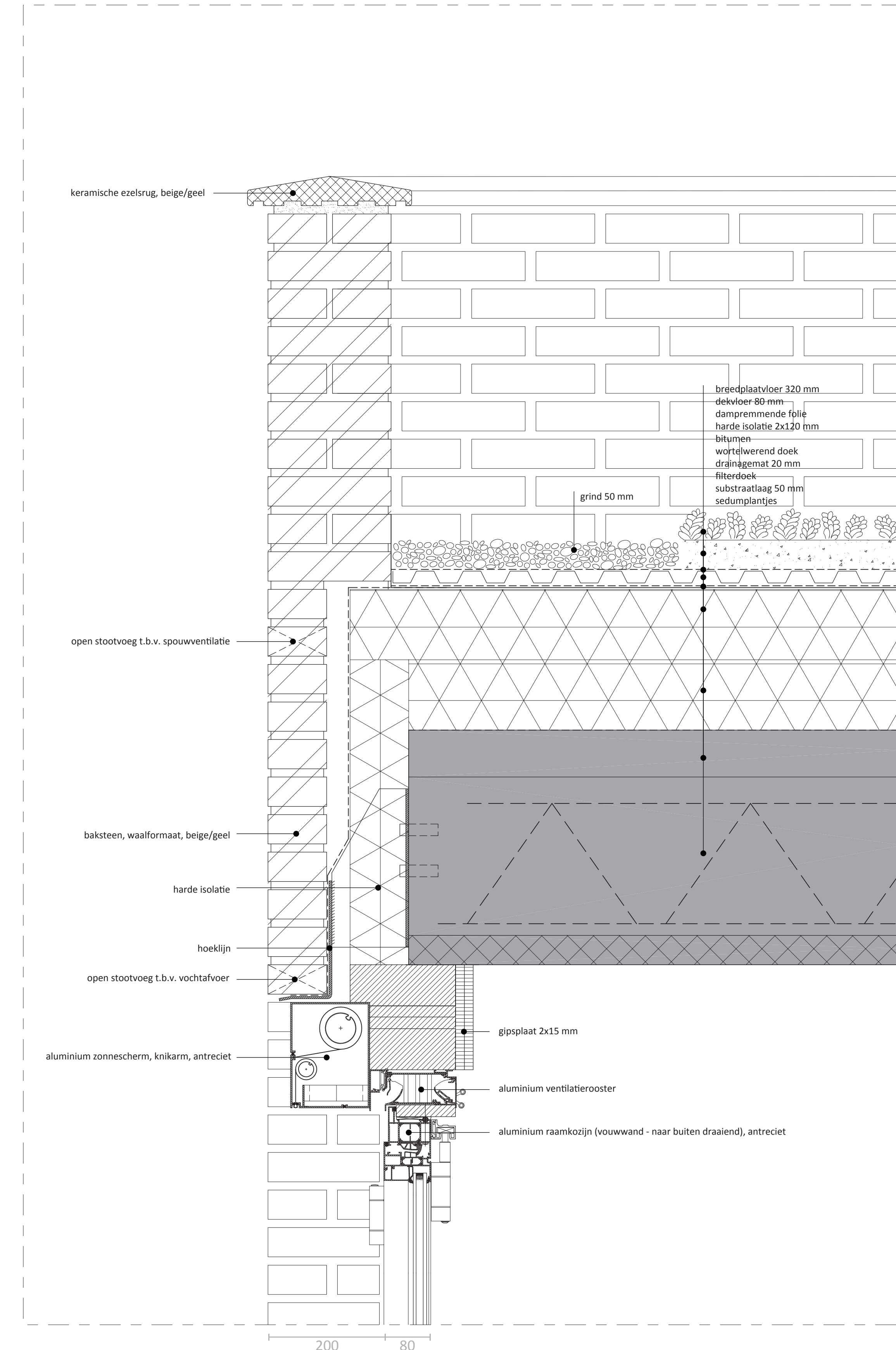
V2: aansluiting kozijn onderzijde (balkon)
