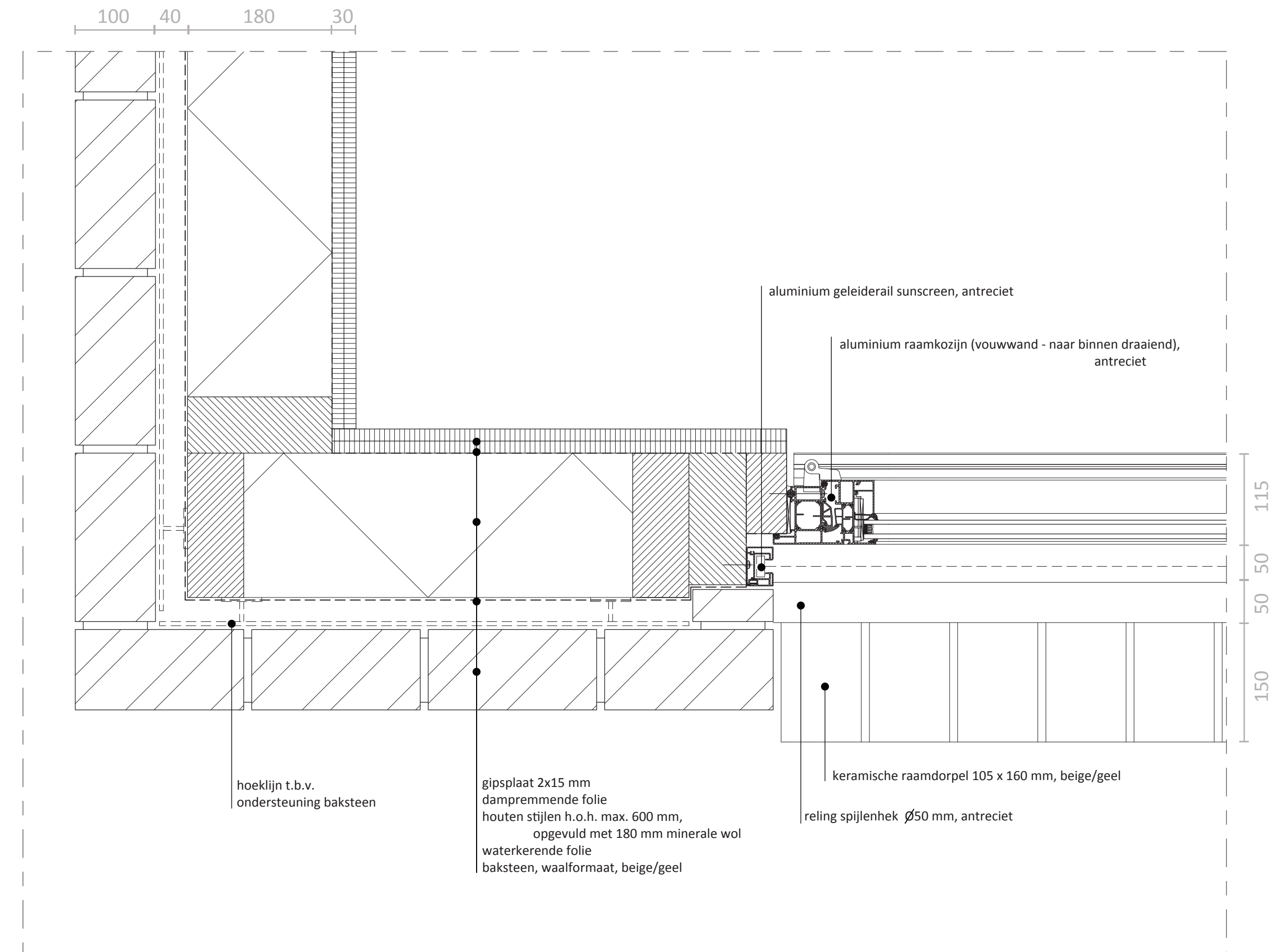
H1: aansluiting kozijn
