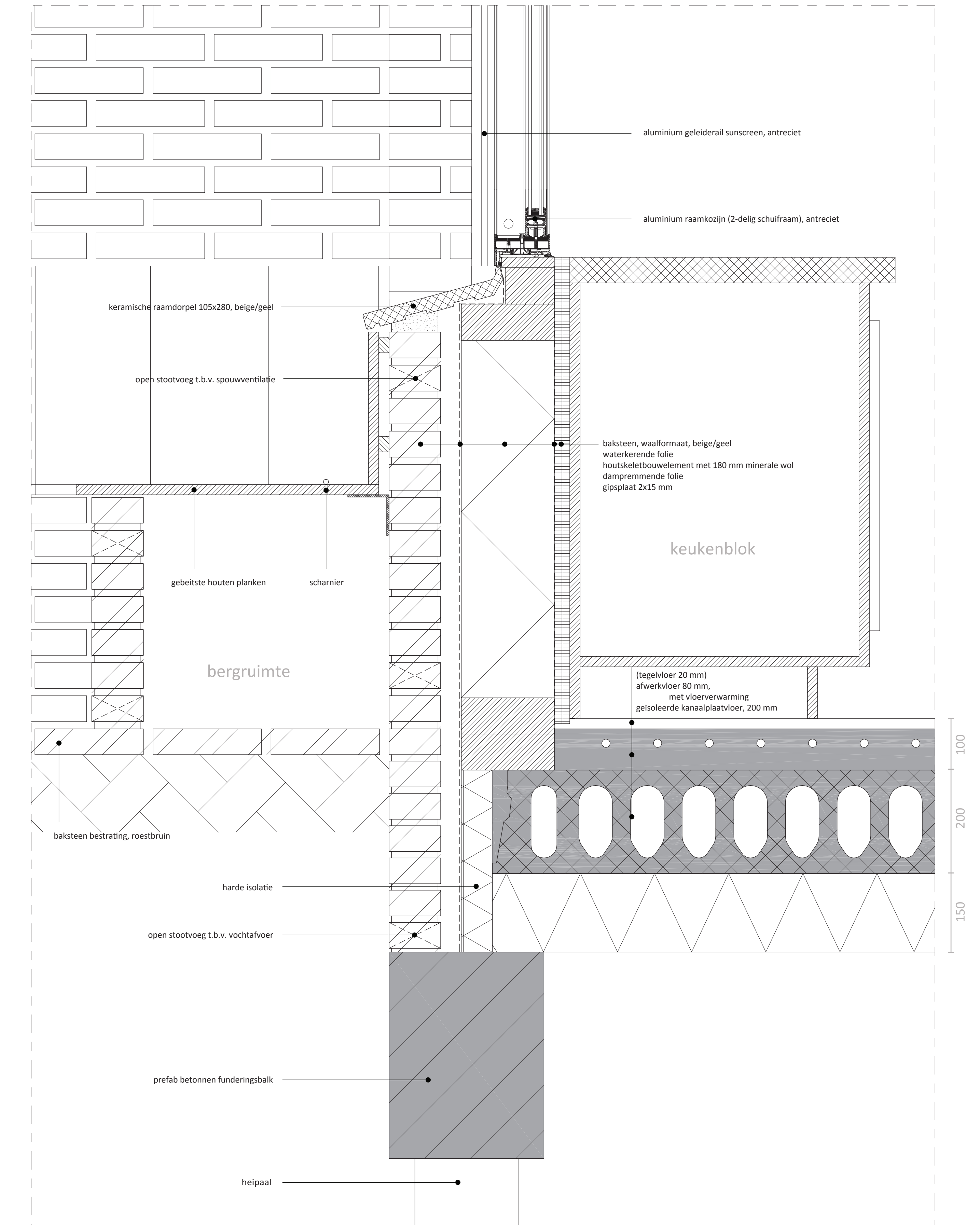
V5: aansluiting kozijn onderzijde - aansluiting fundering
