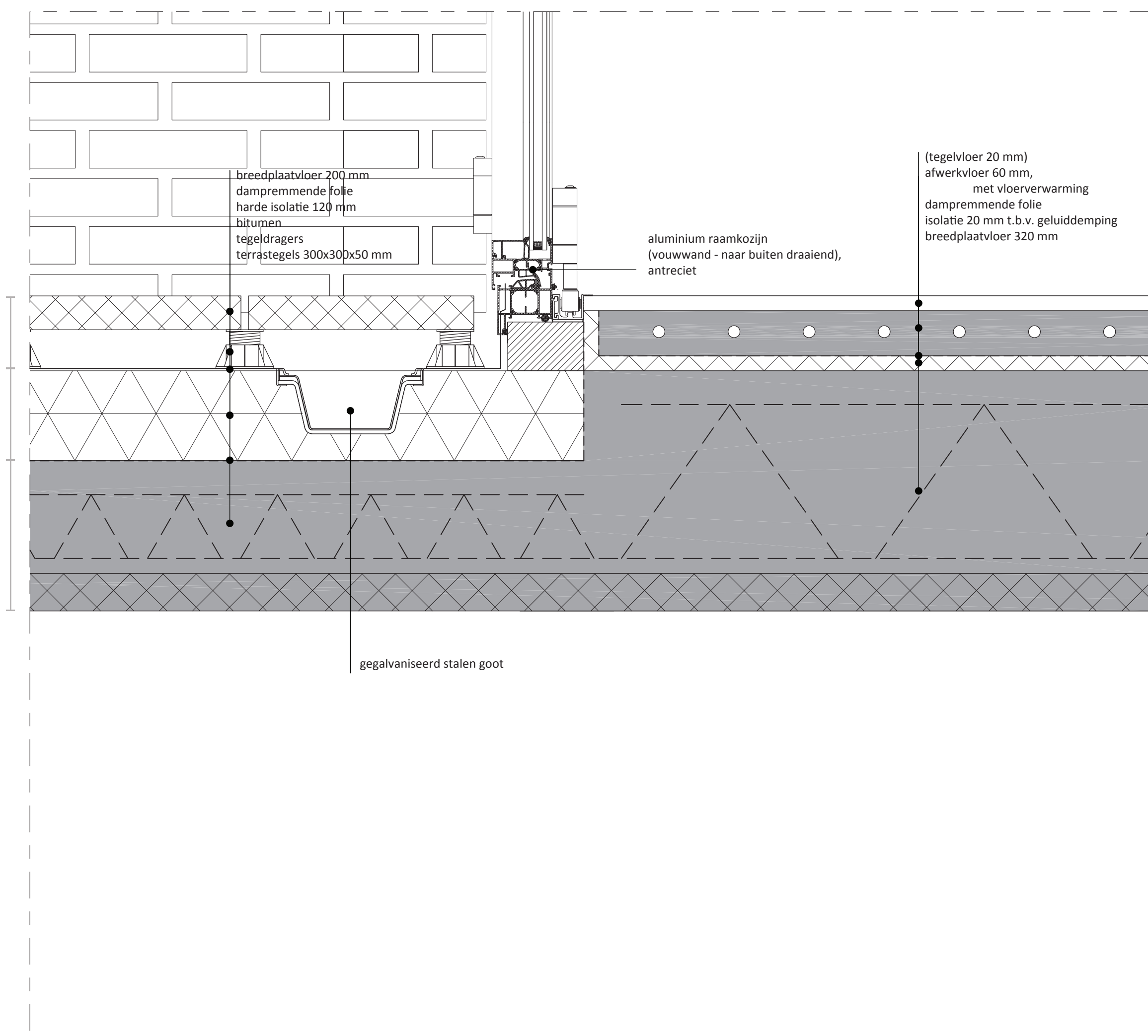
V2: aansluiting kozijn onderzijde (balkon)
