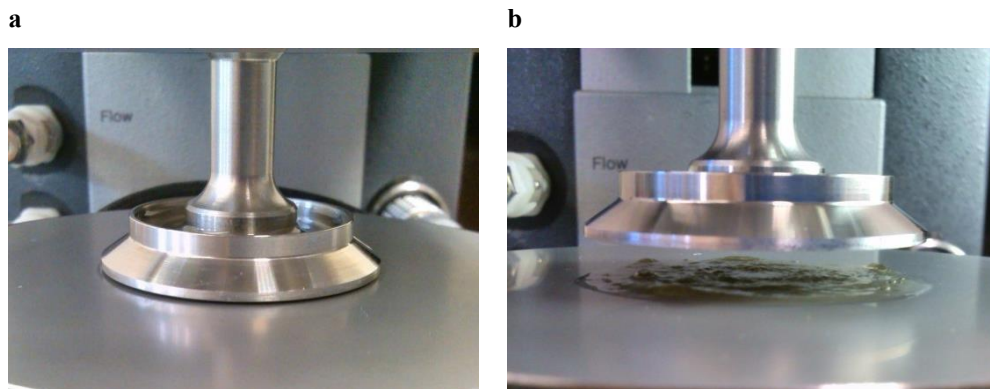
Figuur 4: De rheometer. Het mengsel waarin de gel vormt wordt op de onderste plaat gegoten. De bovenste plaat ligt op de gel en oscilleert zachtjes. De kracht waarmee het materiaal het oscilleren tegenwerkt is een maat voor de stijfheid van de gel. (a) De rheometer in gebruik. (b) De gel is gevormd op de rheometer.
