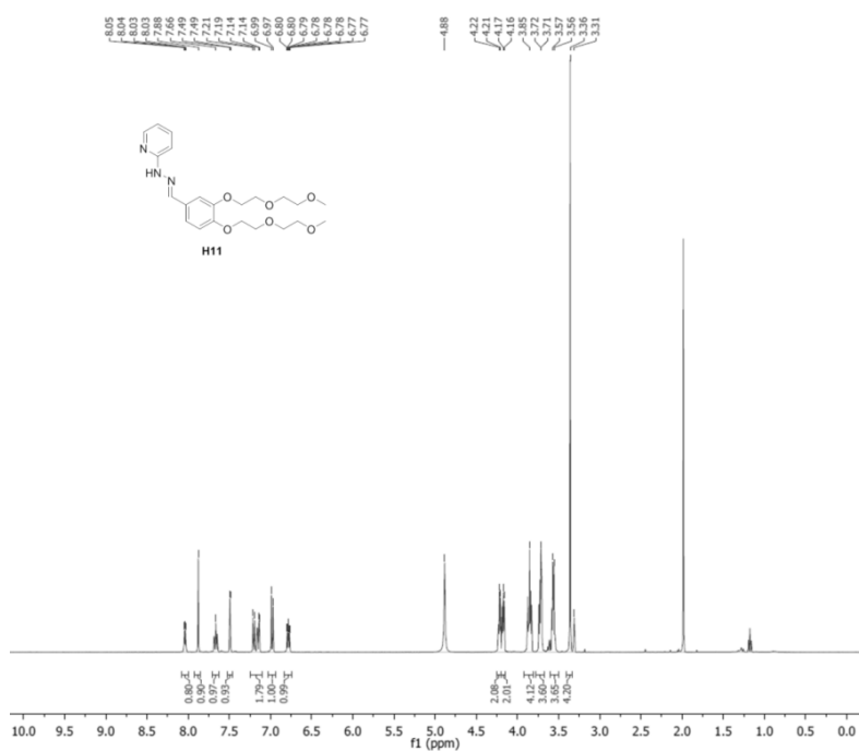
1 H NMR H11 in CD 3 OD
