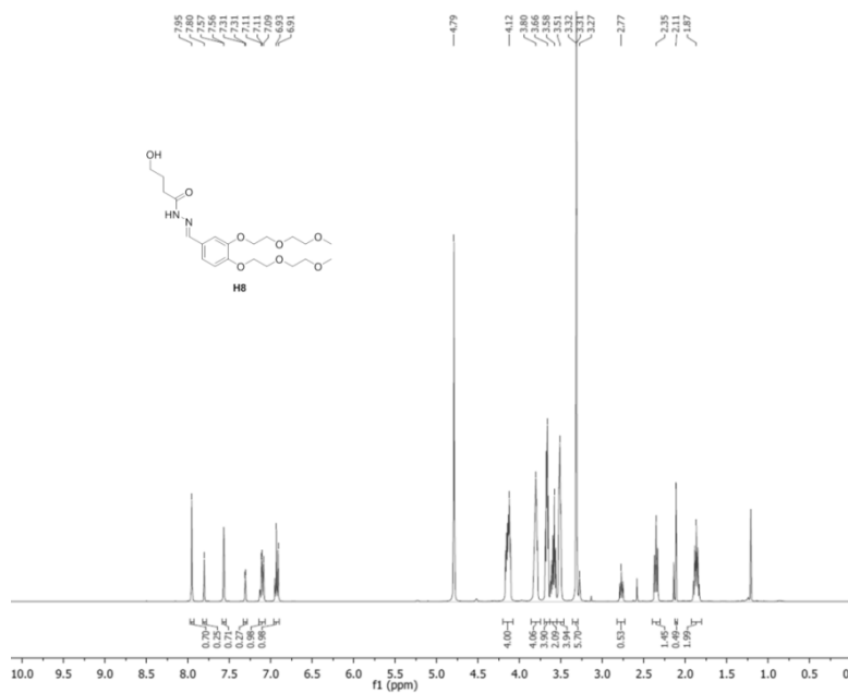
1 H NMR H8 in CD 3 OD
