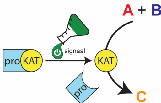
Figuur 2: Een pro-katalysator wordt geactiveerd met een signaal en kan dan een chemische reactie katalyseren.
