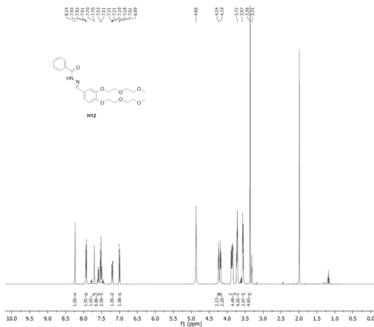
1 H NMR H12 in CD 3 OD
