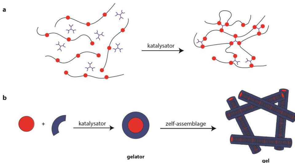
Figuur 1: Hydrogel netwerken. (a) Een polymeergel die covalente cross-links aangaat en op die manier een gelnetwerk vormt. (b) Twee wateroplosbare stoffen reageren met elkaar onder invloed van een katalysator en vormen een gelator. Deze gelator stapelt zich op en vormt zo een gelnetwerk.
