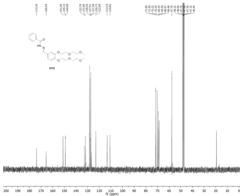
13 C NMR H12 in CD 3 OD
