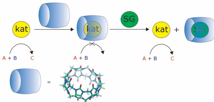
Figuur 5: Cucurbituril (CB) bindt aan katalysator 1 en hindert daarmee de katalyse. Als we een sterker bindende gast, de supergast (SG) toevoegen dan neemt die de plek in van de katalysator, zodat de katalysator weer beschikbaar is om de reactie te katalyseren.
