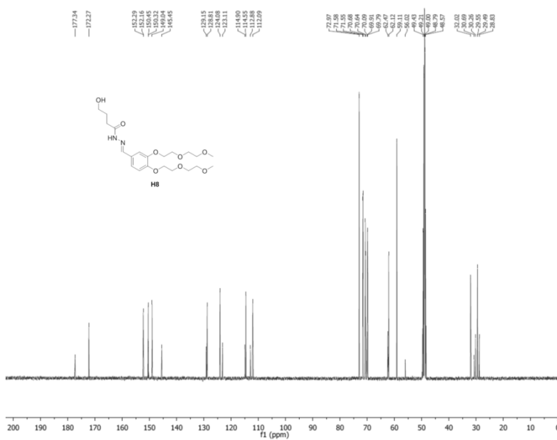
13 C NMR H8 in CD 3 OD
