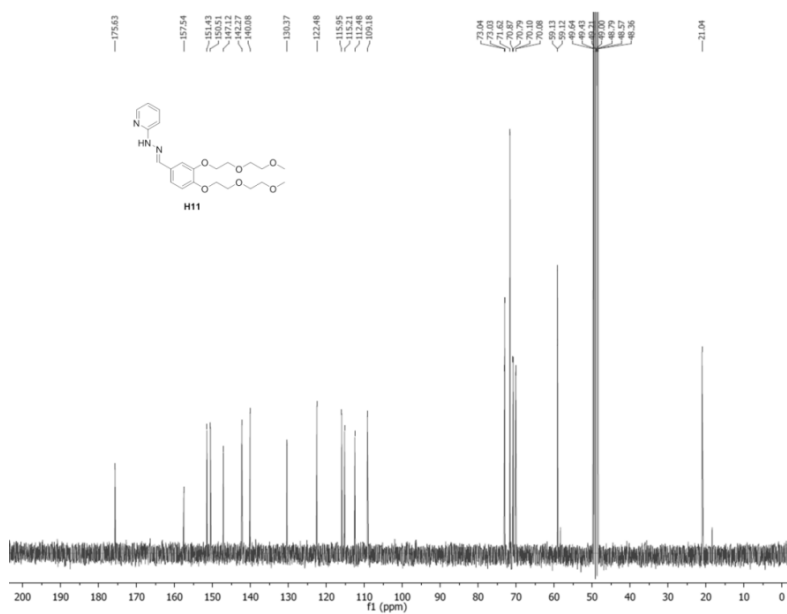
13 C NMR H11 in CD 3 OD
