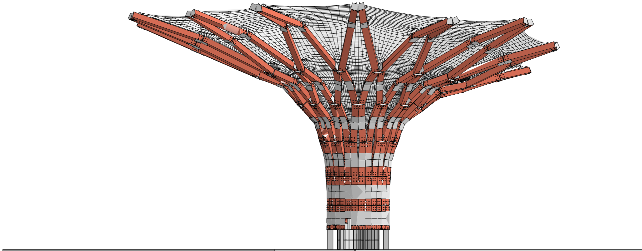
elevation : column : unfolded : 1:100
