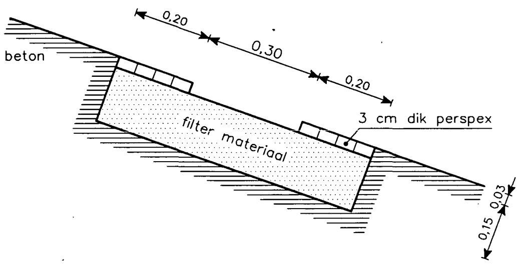
DOORSNEDE A-A
