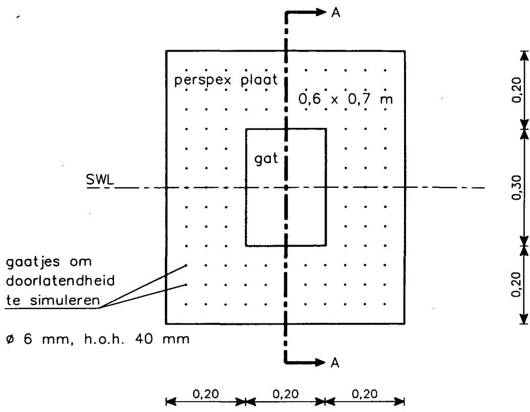
BOVENAANZICHT
