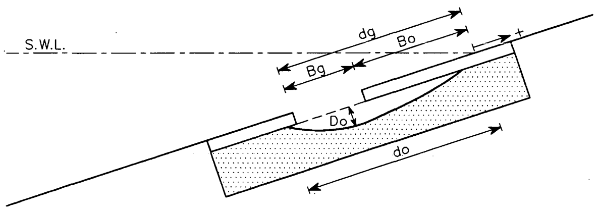
zijaanzicht
