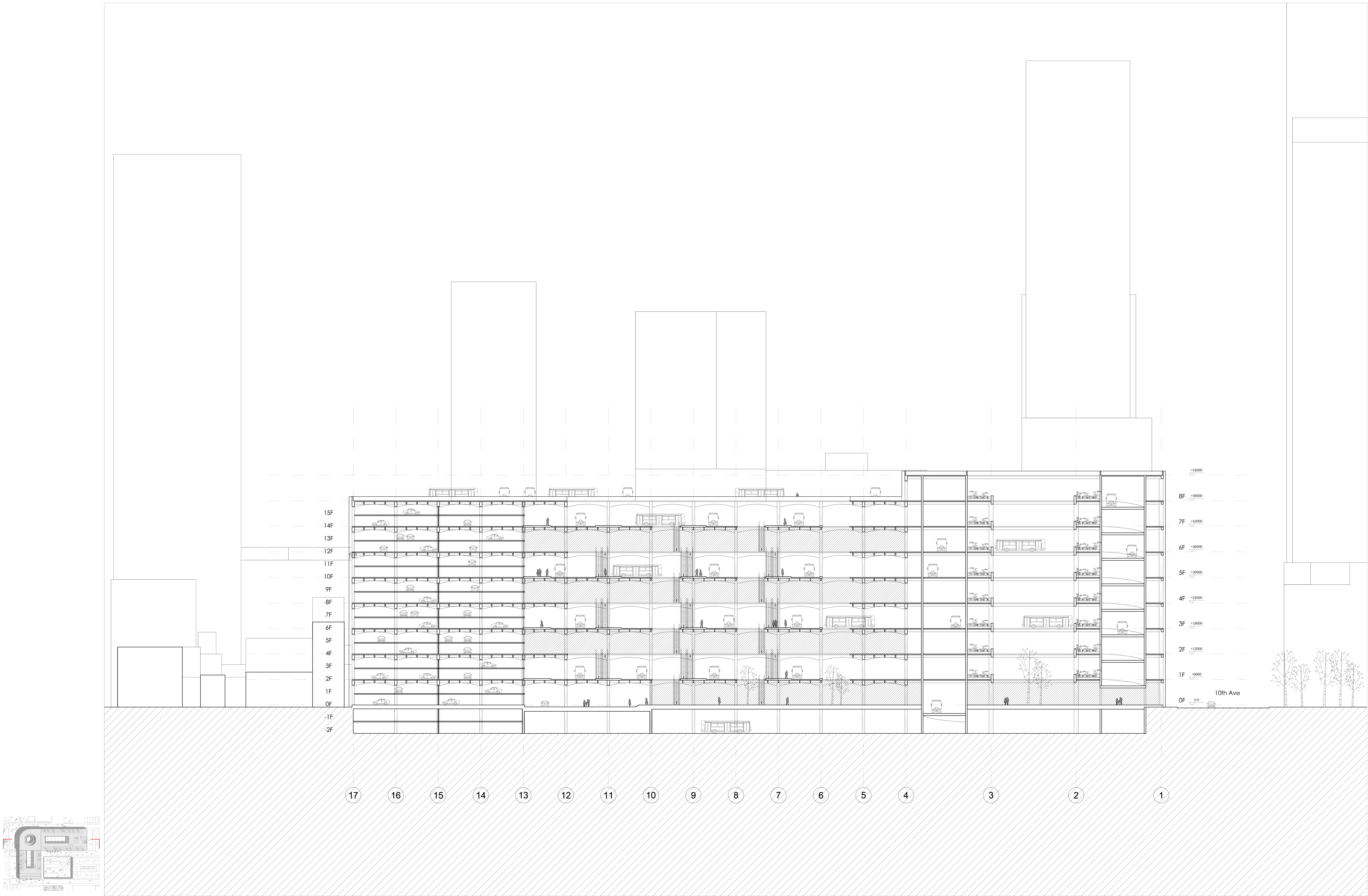
SECTION A-A 1:300
