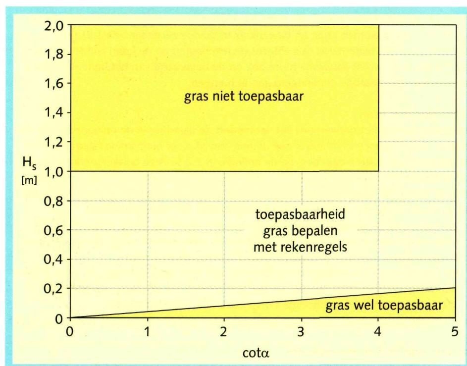
Figuur 4.1 Toepasbaarheid grasbekledingen in de golflapzone
