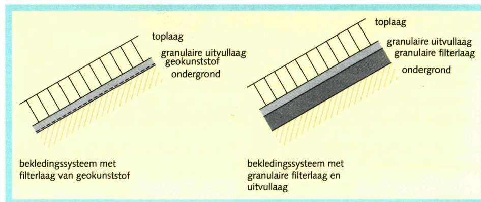
Figuur 2.6 Twee typen filters
