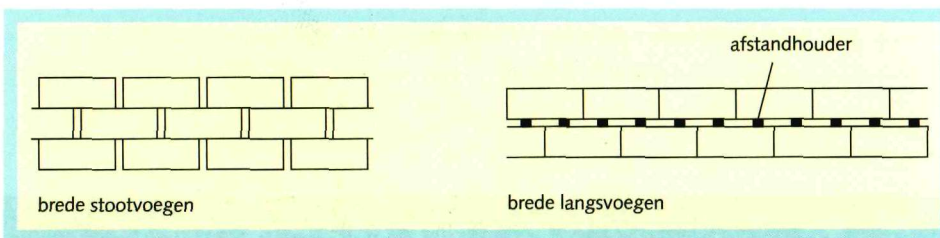
Figuur 2.2 Twee maatregelen ter vergroting van de open ruimte (bovenaanzicht)
