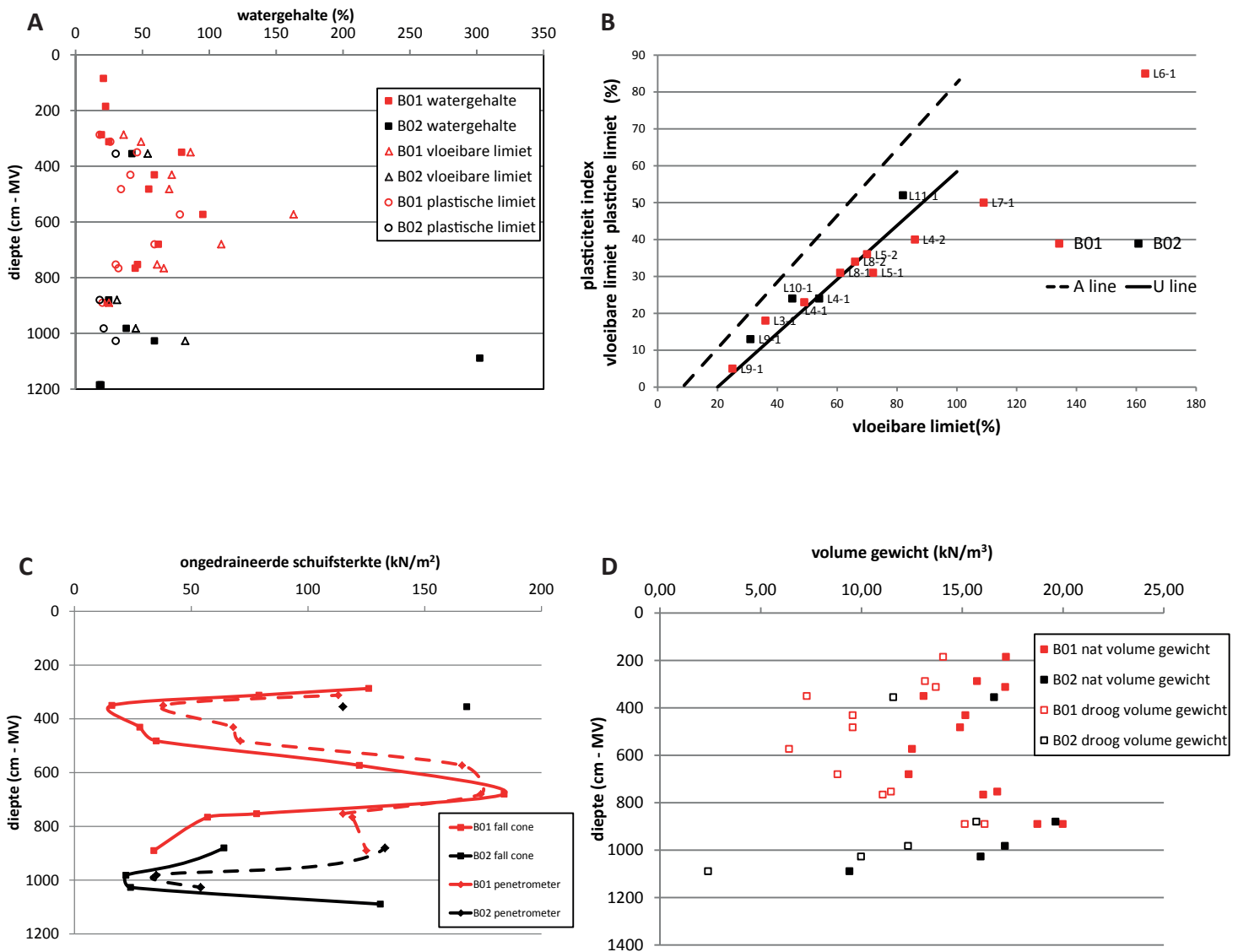
Fig. 56 Geotechnische resultaten. A: verloop van watergehalte, vloeibare limiet en plastische limiet per diepte. B: plasticiteits grafiek. Alle monsters plotten onder de A-lijn en de meeste monsters iets boven de U-lijn. De U-lijn is de bovengrens van de relatie tussen de plasticiteitsindex en de vloeibare limiet voor natuurlijke gronden; de A-lijn scheidt anorganische kleien van anorganische silten en organische gronden. De monsters uit Hogebeintum kunnen op basis van deze figuur worden geclassificeerd als kleien of organische kleien. C: Ongedraineerde schuifsterktewaarden per diepte, geschat met de vallende kegel en de hand-penetrometer. De waarden zijn verschillend maar volgen dezelfde trend. D: variatie in volumegewichten per diepte. Figuur D. Ngan-Tillard.
