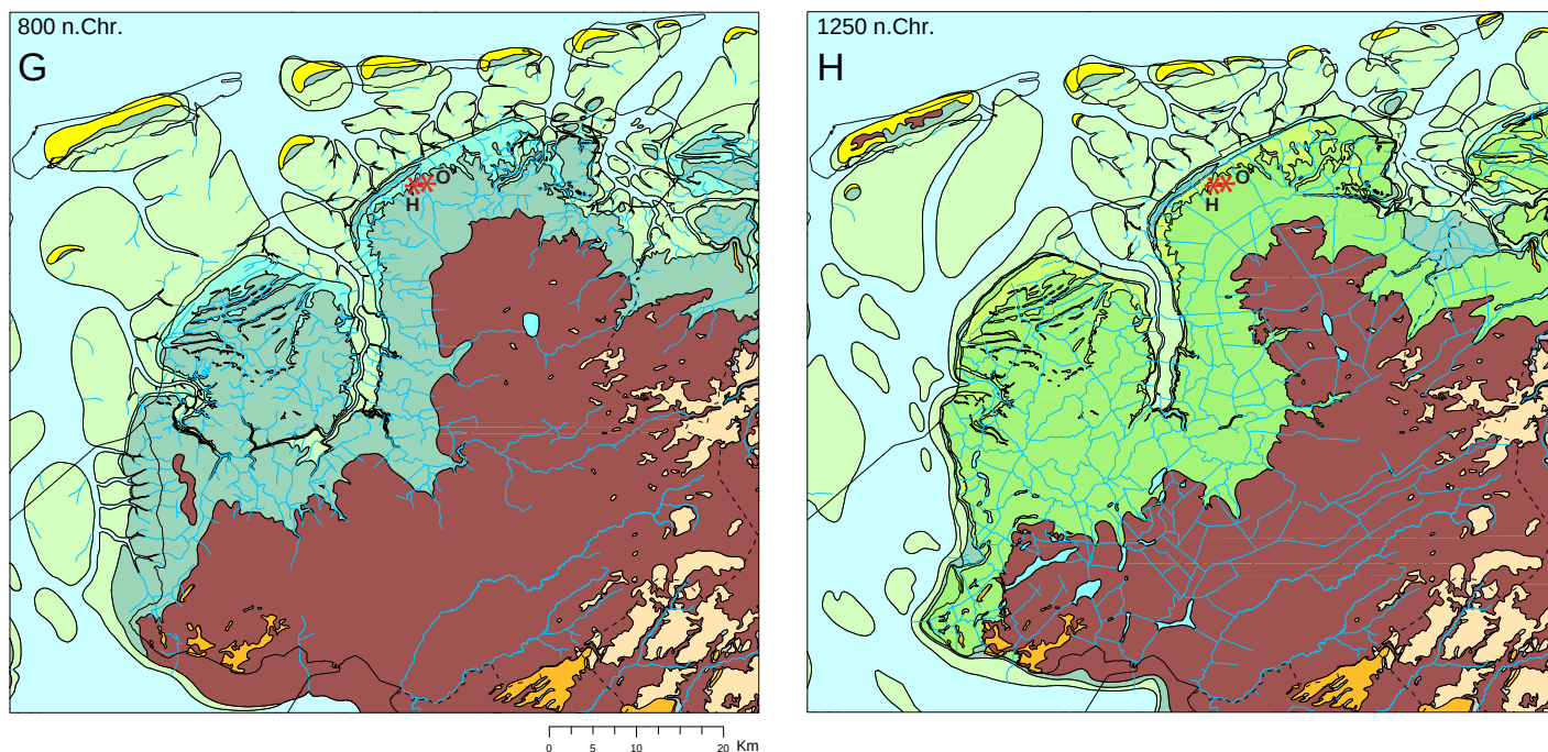
Fig. 19 Palaeogeografische kaarten van Friesland, voor acht perioden, van 3850 v.Chr. tot 1250 n.Chr. (A tot H). De locaties van Hogebeintum (H) en Oosterbeintum (O) zijn aangegeven. Kaarten P.C. Vos & S. de Vries, Deltares.
