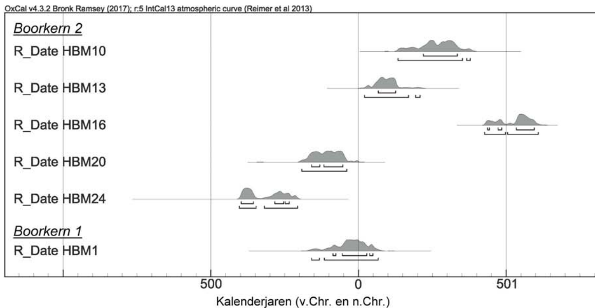
Fig. 22 Overzicht van de ^{14}\text{C} -dateringen van organische monsters uit beide steekboringen, omgerekend in kalenderjaren. Kalibratie met Oxcal v4.3.2, met betrouwbaarheidsintervallen voor 1 en 2 sigma (zie tabel 3). Figuur A. Nieuwhof.
