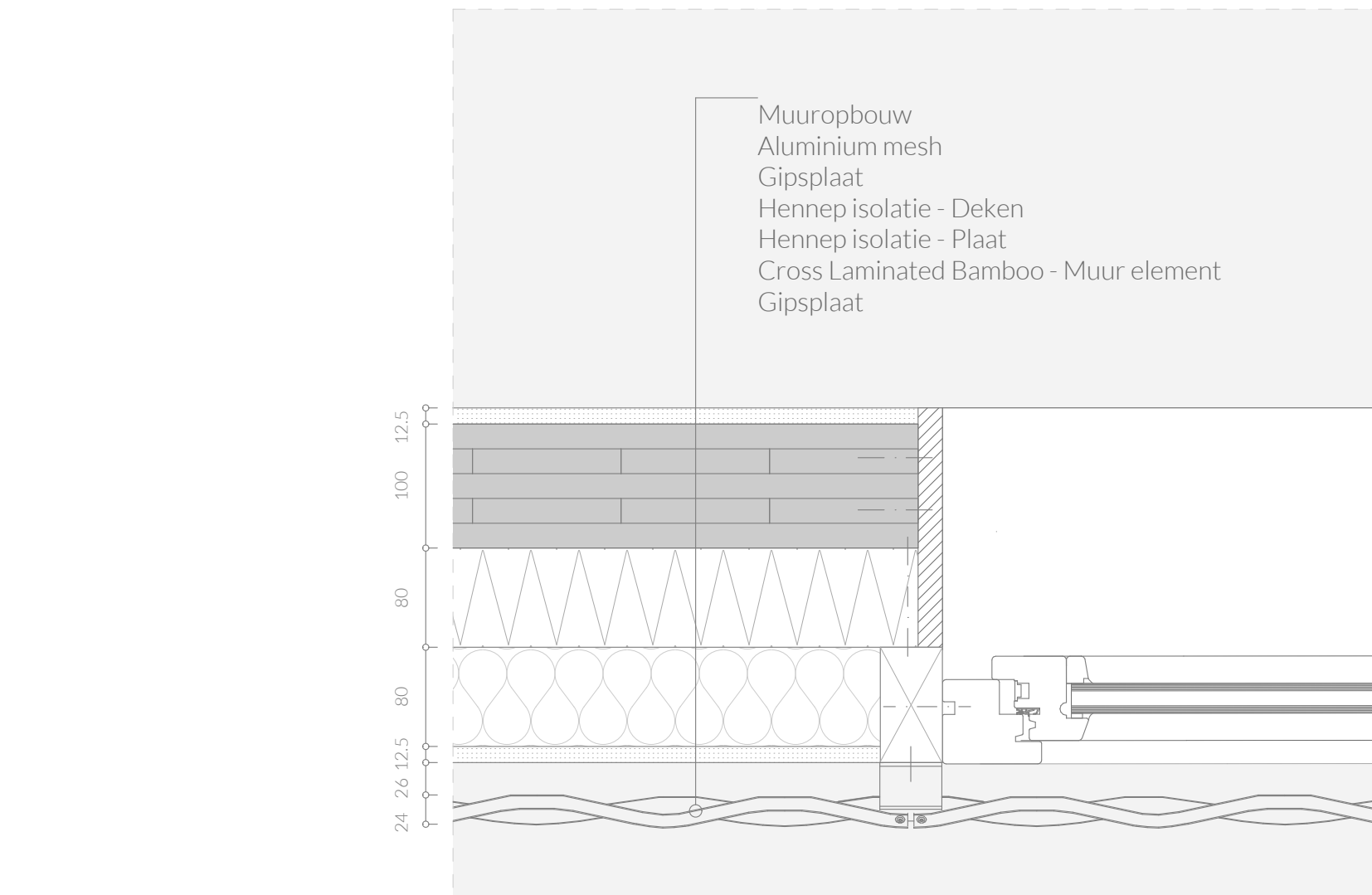
Detail E (horizontaal): Kozijn 1:5
