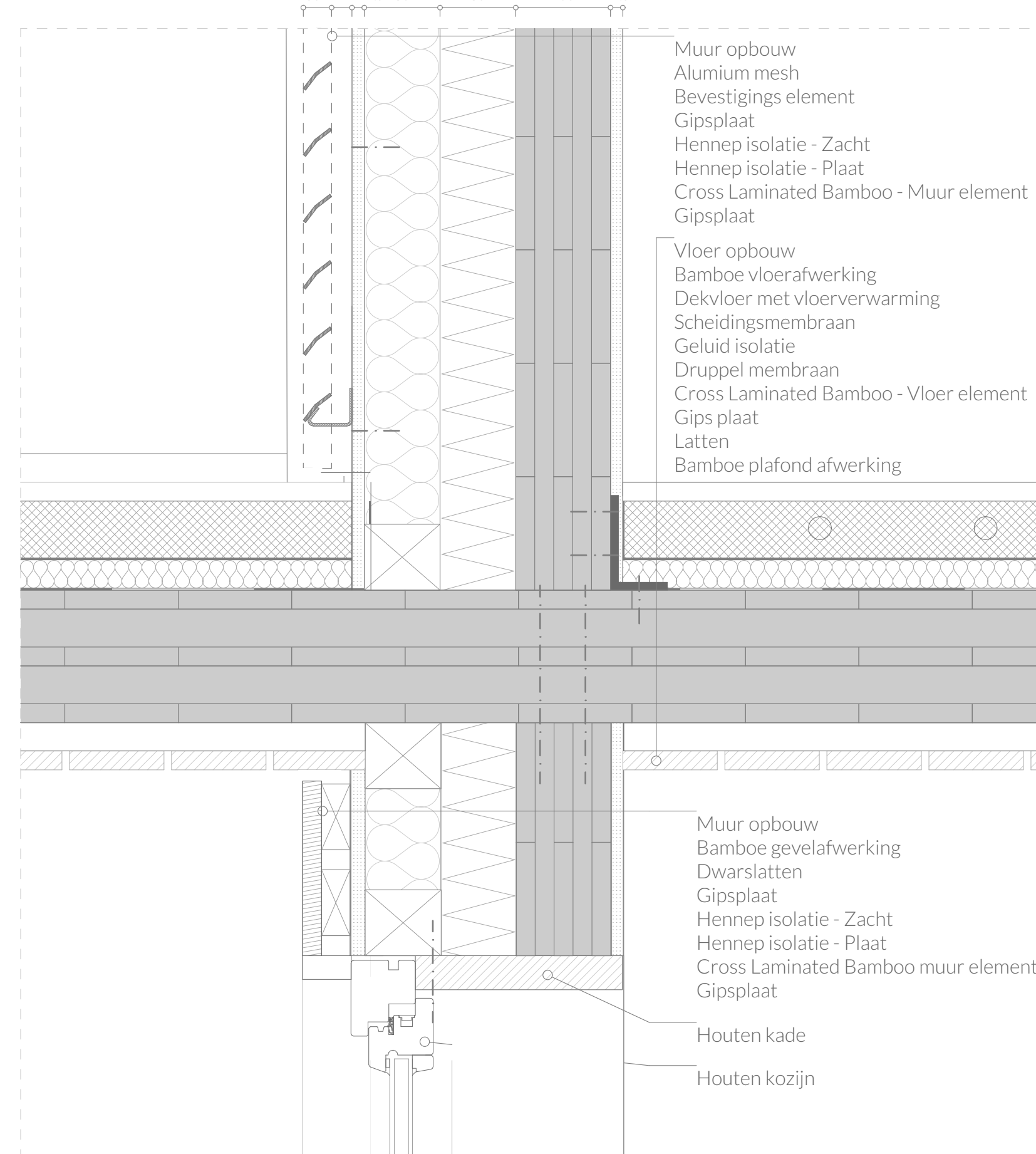
Detail B: Verdiepingsvloer 1:5
