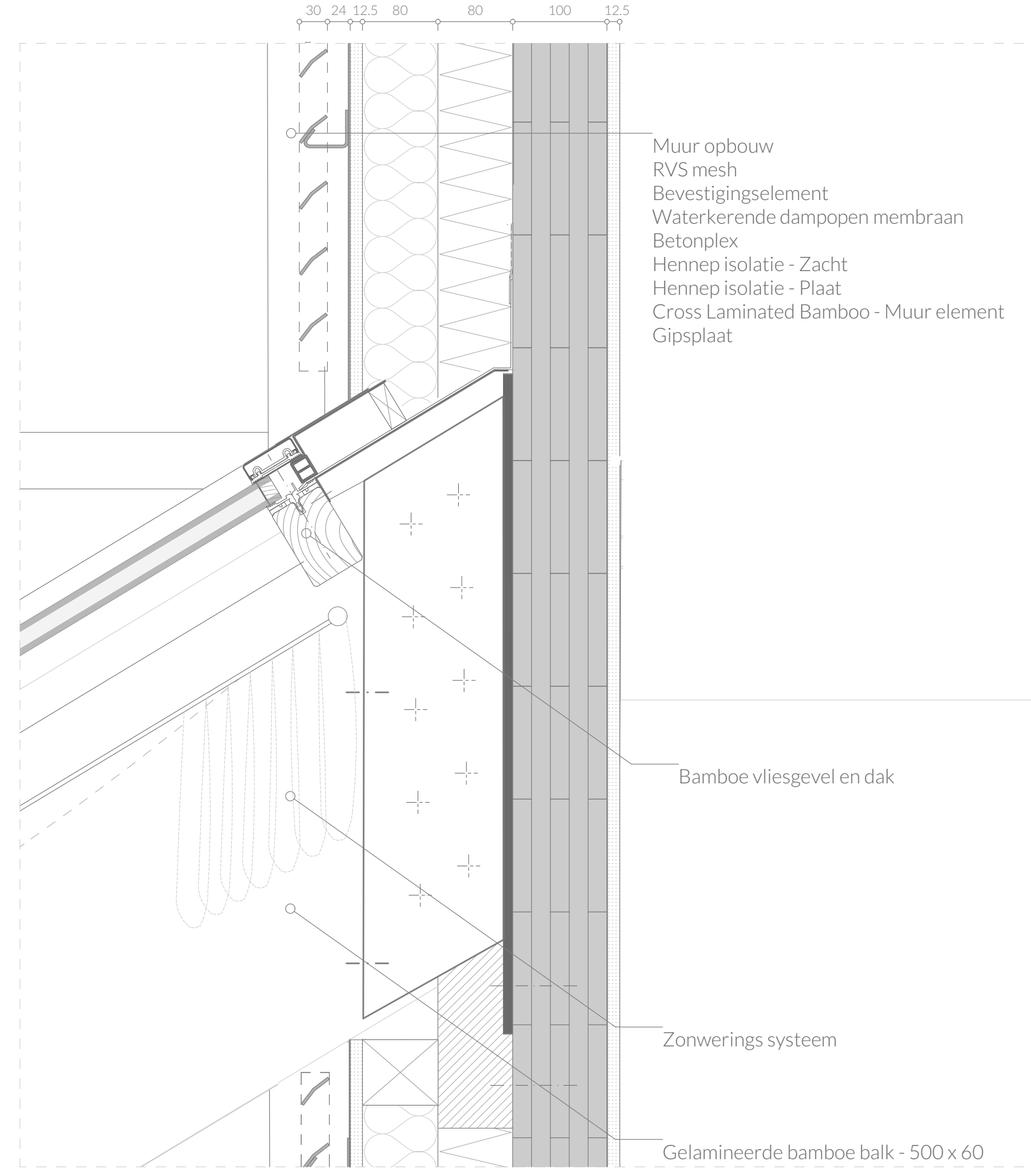
Detail C: Glasdak aansluiting 1:5
