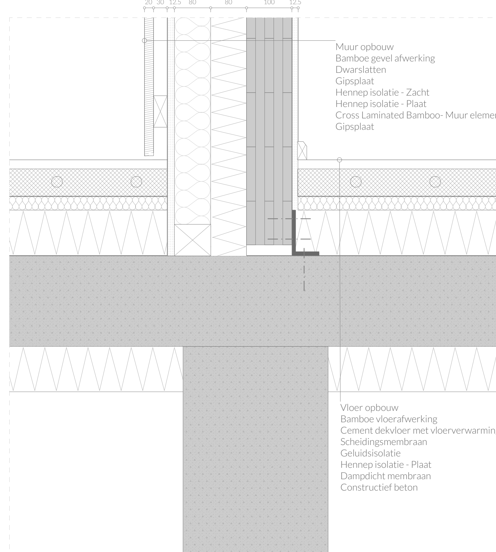
Detail A: Fundering 1:5
