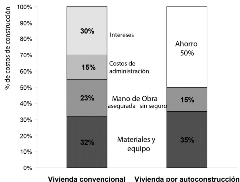
Figura 3. Costos de construcción relativos de vivienda convencional y por autoconstrucción. (Fuente: Mangin y Turner, 1968).
