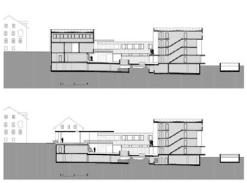
Die Schritte zeigen den integrativen Umgang der Gebäude mit dem Gelände. © Architekten: Rainer Koberl | Daniela Kross
