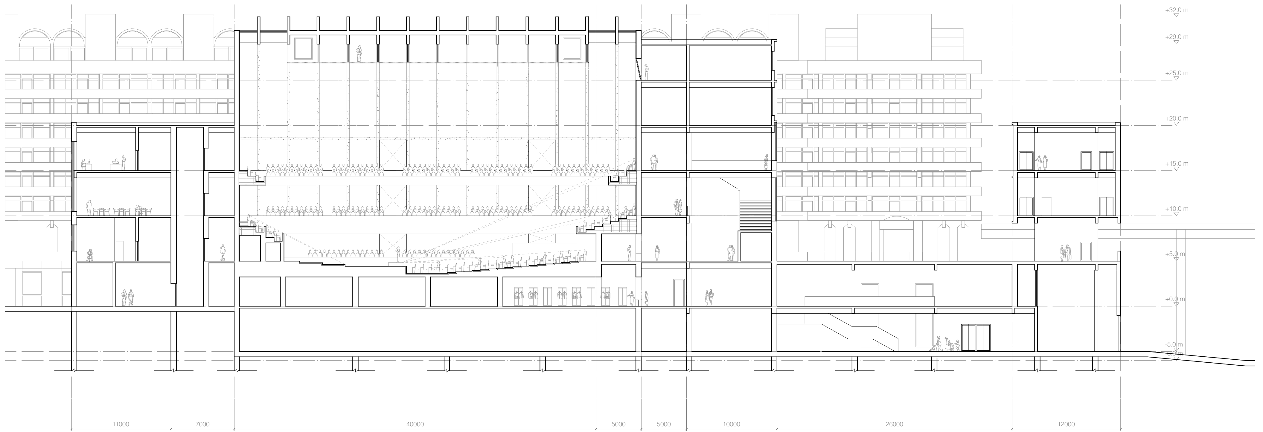
Section BB' 1:250
