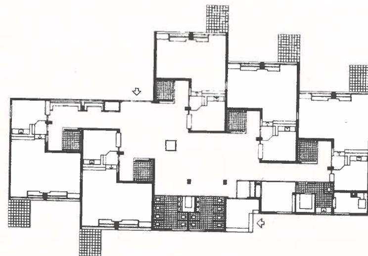
图 13: 代尔夫特蒙特特利学校的原平面图，1960 年设计
