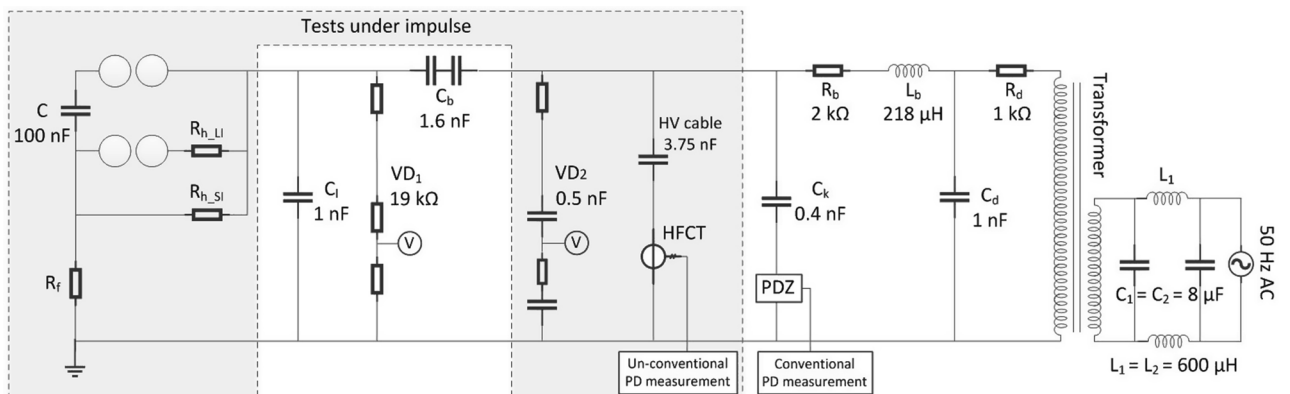
Fig. 1. Test circuit.
