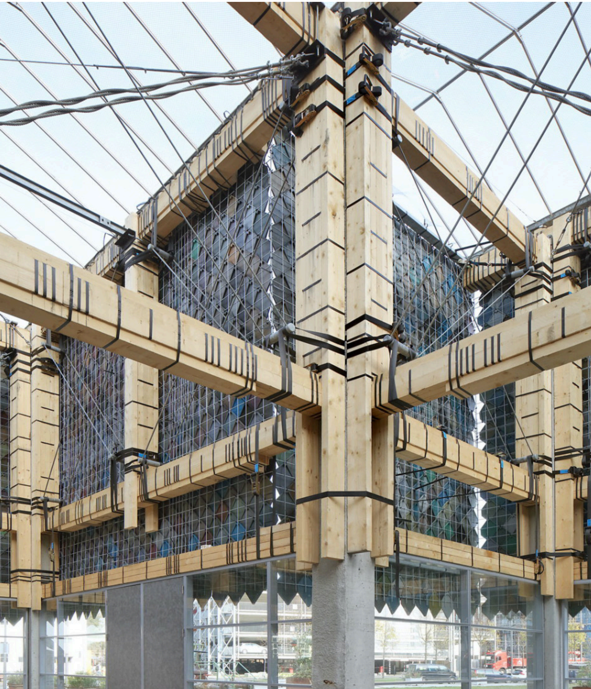
Houtconstructie met spanbanden bevestigd aan betonnen kolommen Referentie: Peoples Pavilion - Bureau SLA - Foto: Filip Dujardin (2017)
