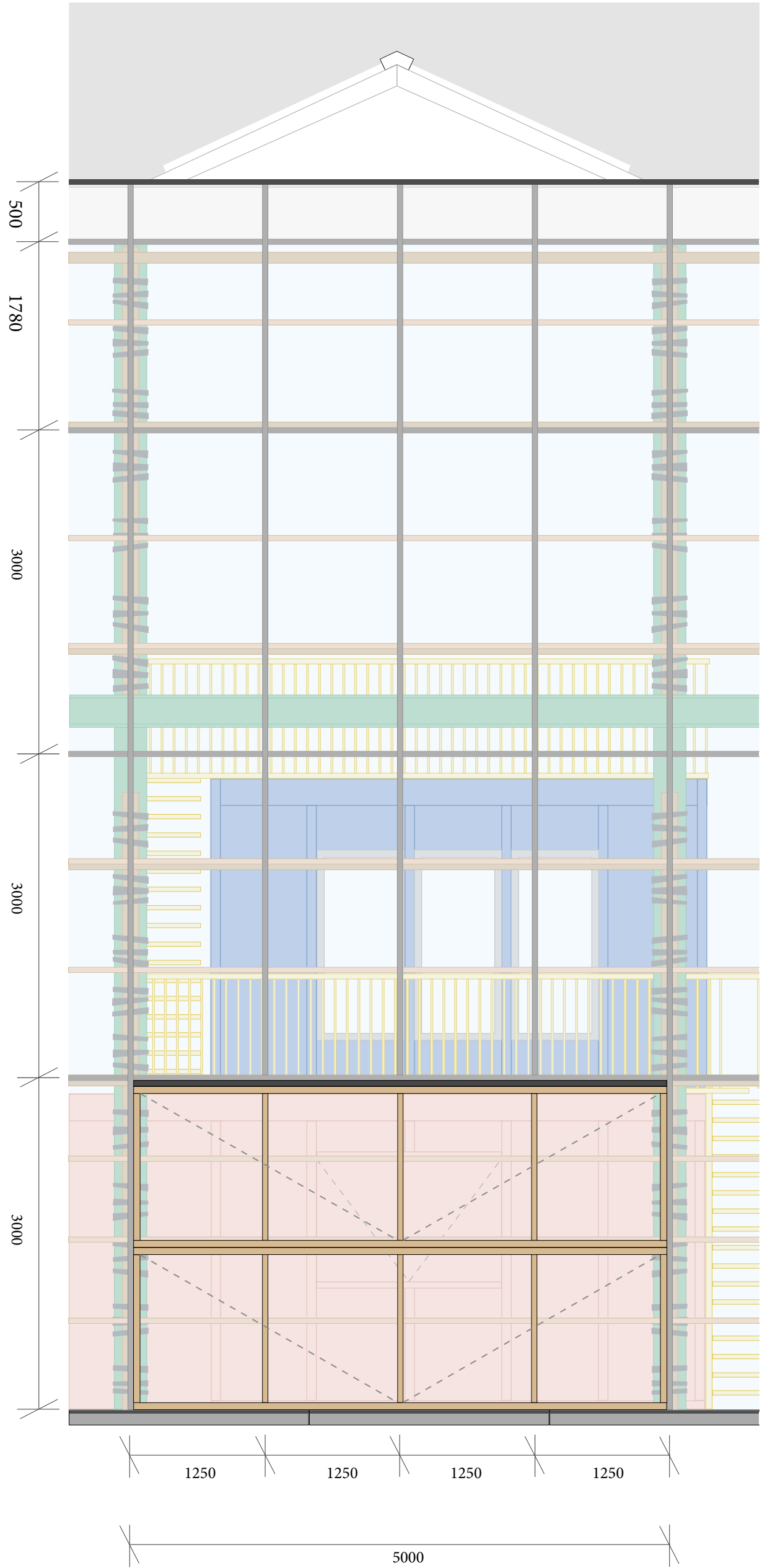
Detail 1:20 en sfeerbeeld
