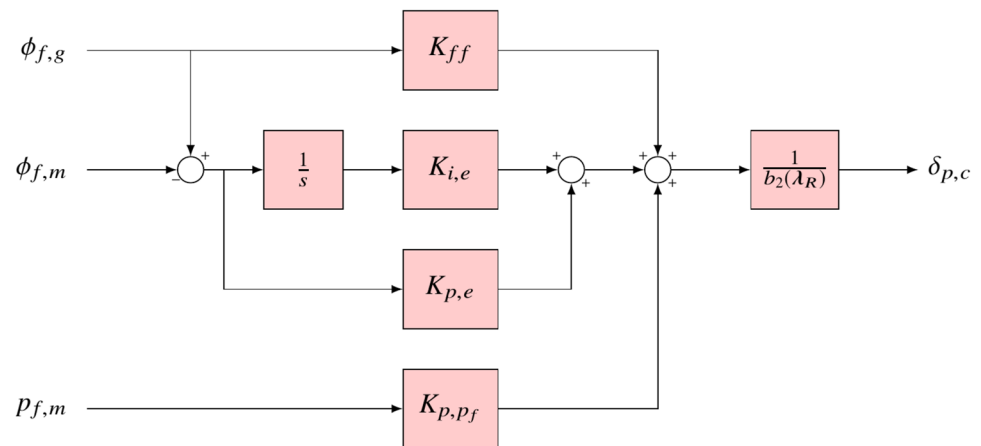
Fig. 4 Roll autopilot structure
