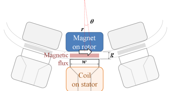
Fig. 1 EM spring concept
