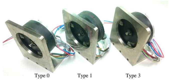
Fig. A1 Three EM spring VSA prototypes.
