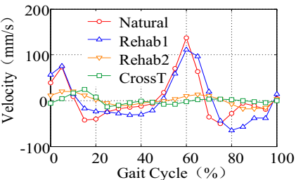
(b2) Comparison of Tibialis Anterior velocity
