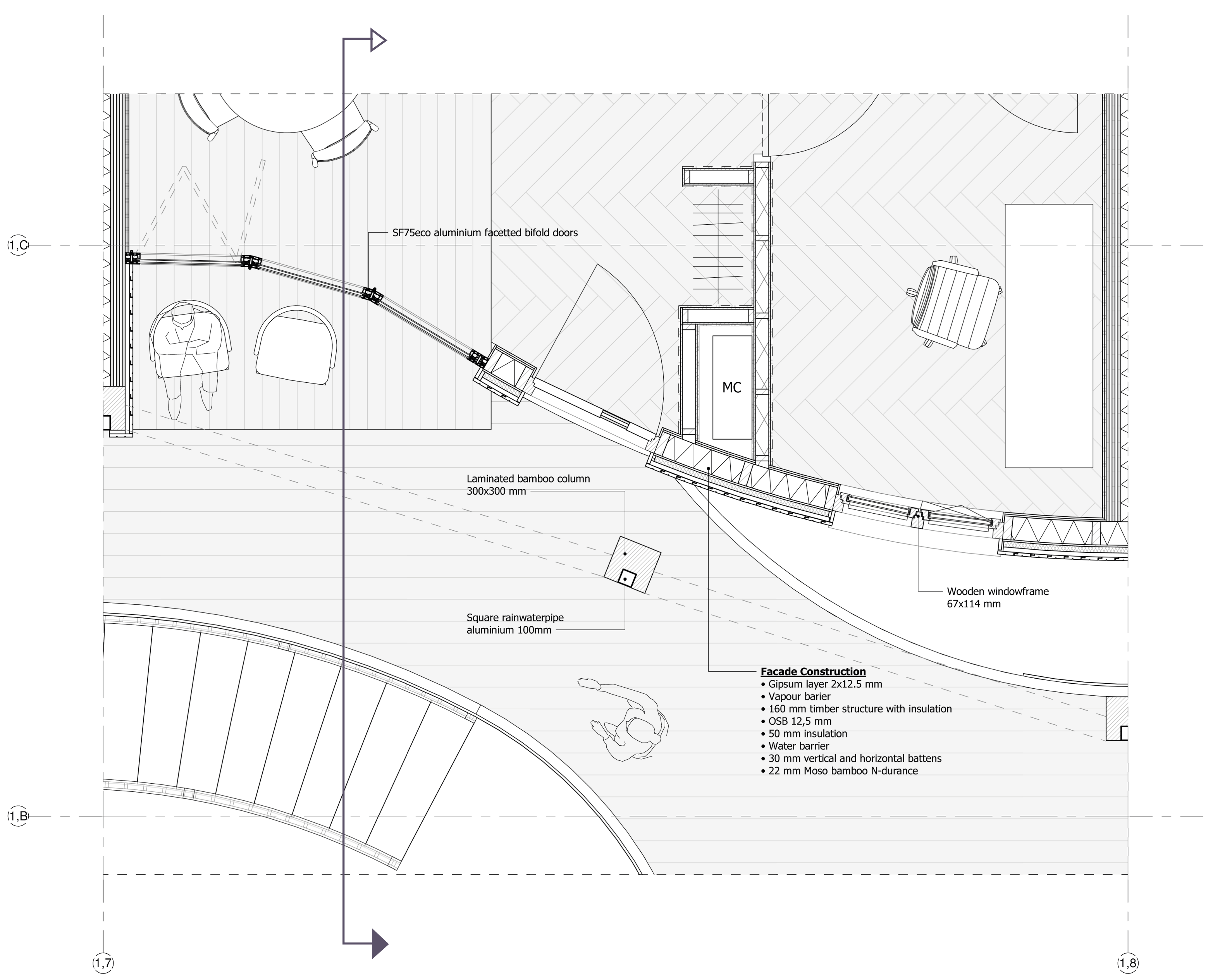
PLAN FRAGMENT 1:20
