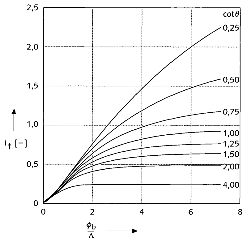
Figuur 5.1 Rekenregel voor het opwaarts verhang i_{\uparrow}
