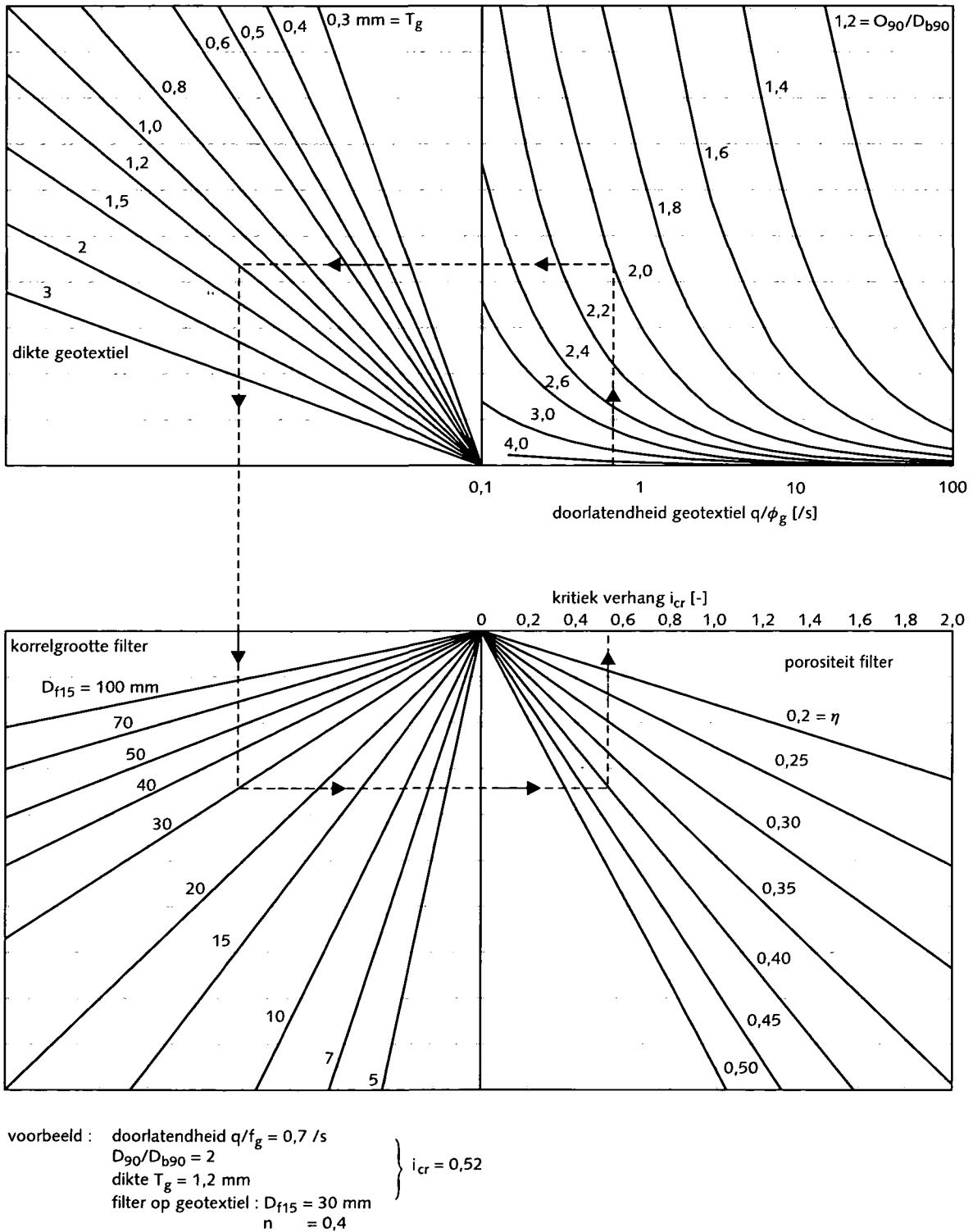
Figuur 5.6 Rekenregel voor het kritiek verhang i_{cr} bij granulaire filter op zand
