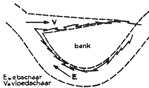
Fig. 13 Schema van de werkelijke zandbeweging bij een veel voorkomend systeem van eb- en vloedscharen.
