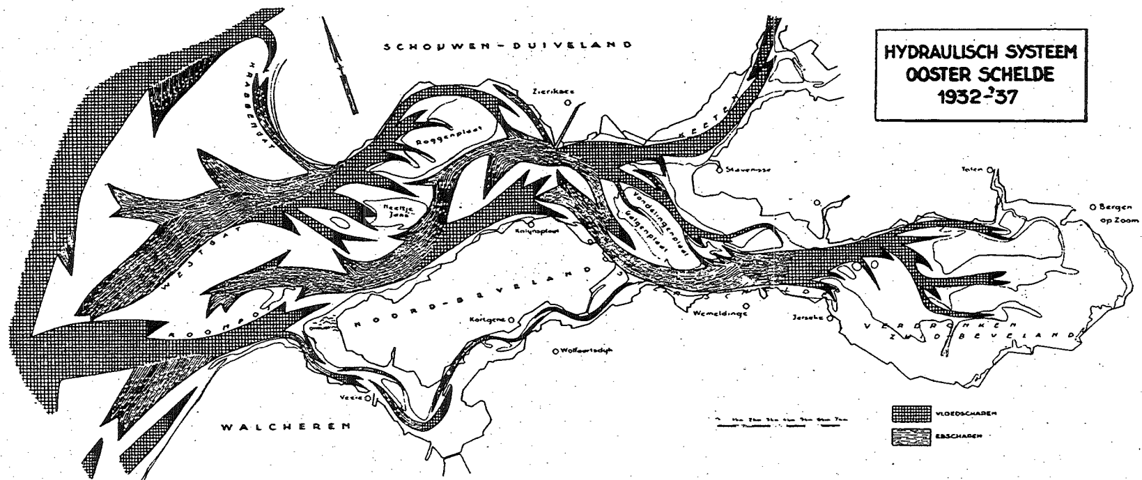
Fig. 29 Systeem van eb- en vloedscharen op de Ooster-Schelde in 1937.
