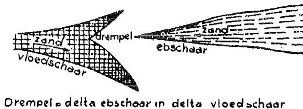
Fig. 10 Schema van het elkaar vermijden van een eb- en een vloed-schaar door middel van vorming.
