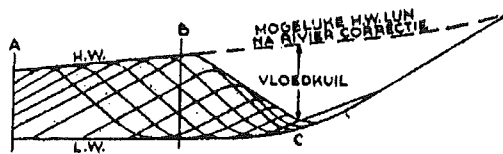
Fig. 7 Verklaring van het begrip vloedkuil.
