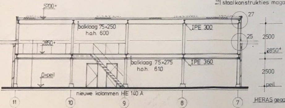
doorsnede F-F (over magazijn)
