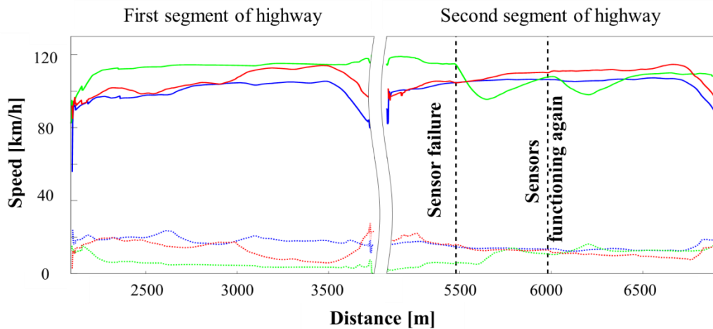
Figuur I.A: Gemiddelde (getrokken lijn) en standaardafwijking (stippellijn) van snelheidsverdelingen berekend als een functie van de afgelegde afstand sinds het begin van de simulatie voor de basislijnvoorwaarde (blauw), de experimentele toestand 1 (groen) en de experimentele voorwaarde 2 (rood).
