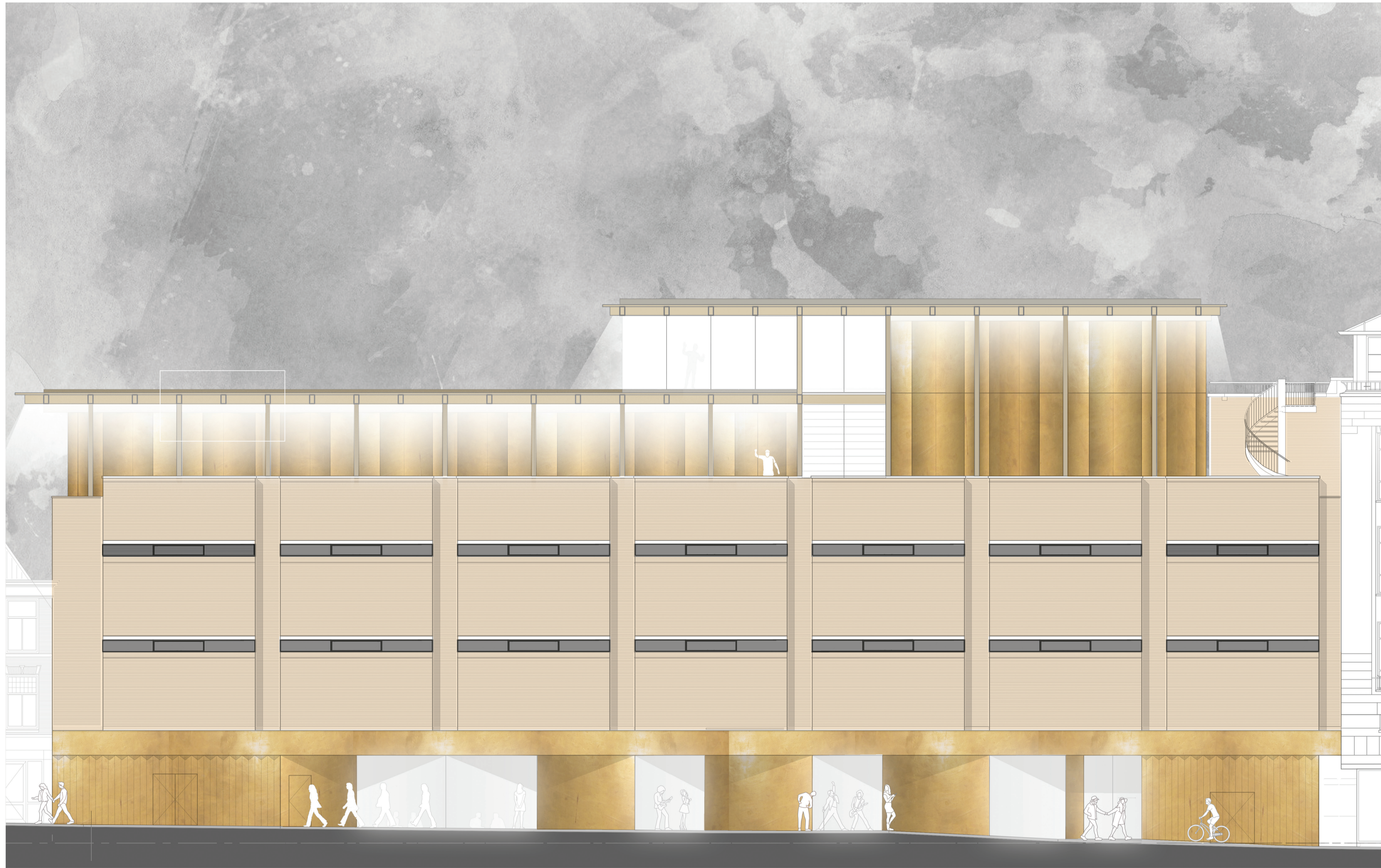
MAARSMANSTEEG ELEVATION
