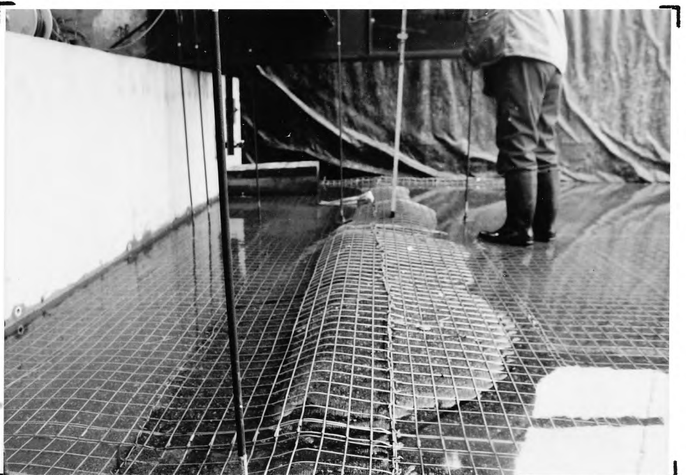
5. Opbollen van de mat \pm 1 m voor de drukbalk.
