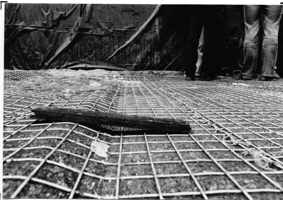
7. Het omhoogkomen van de mat rechts in de proef- bak.
