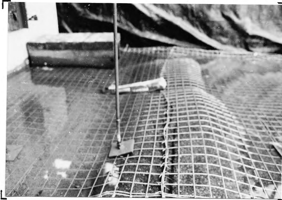
6. 6 Het omhoogkomen van de mat links in de proef- bak.
