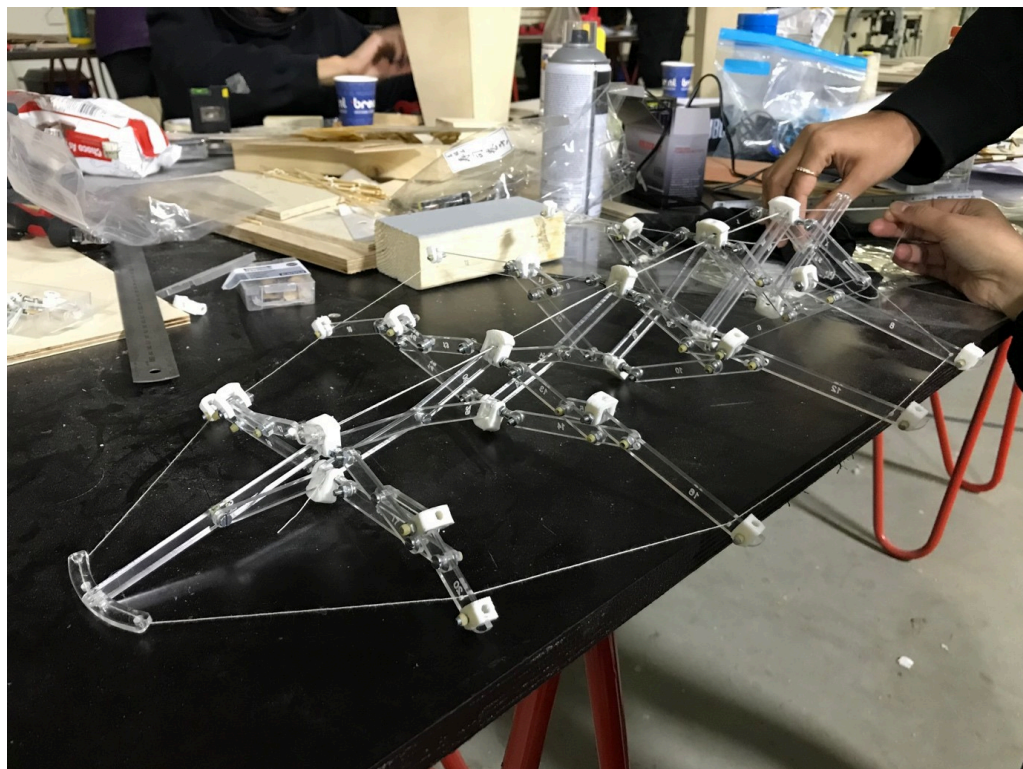
Fig.5 functiemodel van een zonnenuif 1:5 (door Krittika Agarwal, Priyadarshini Nanda, Shweta Kamble, Pierre Kauter en Okan Türkan, gebruik met toestemming).
