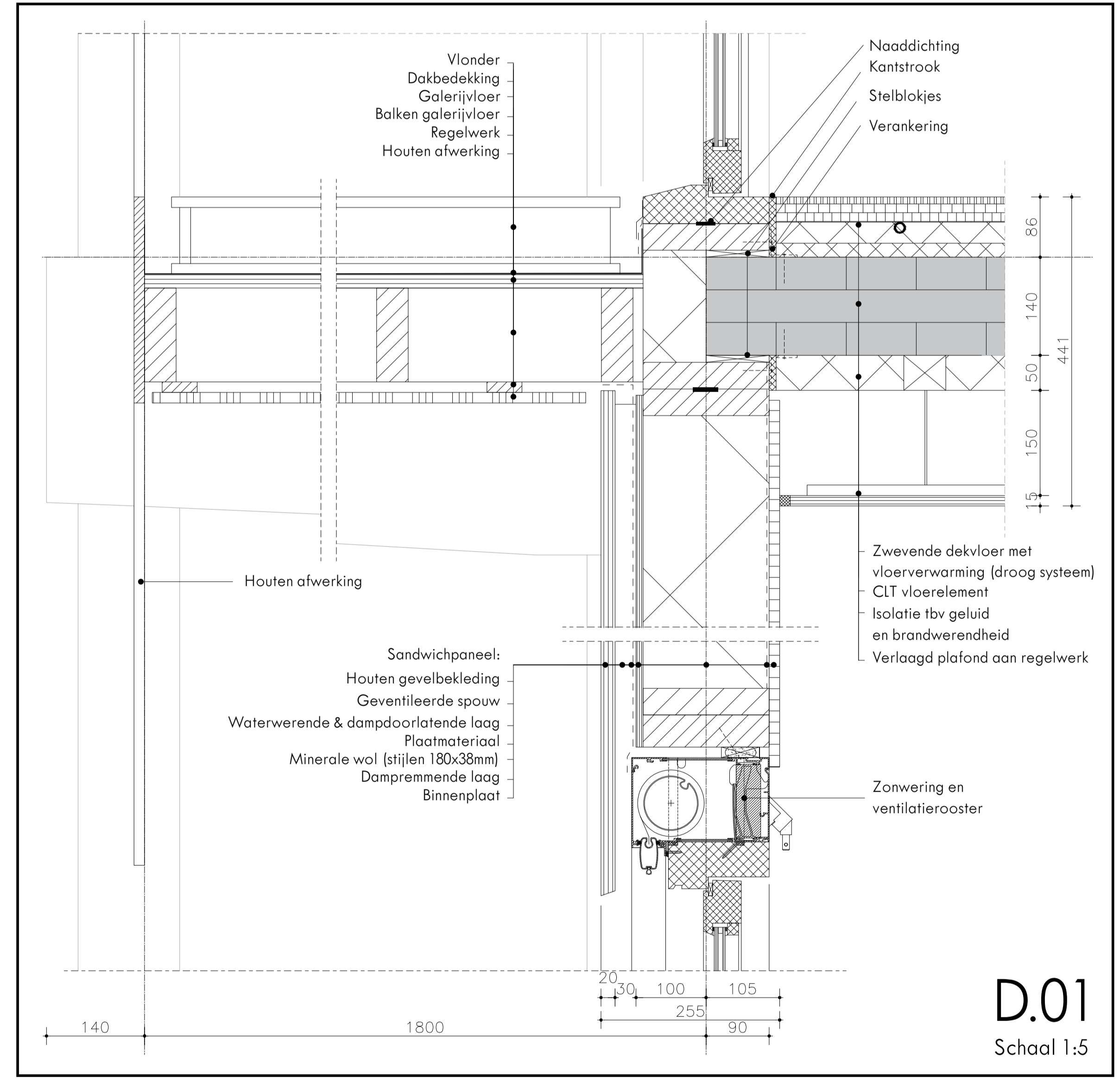
UITWERKING WAND Lengte-, dwars- en horizontale doorsnede wand
