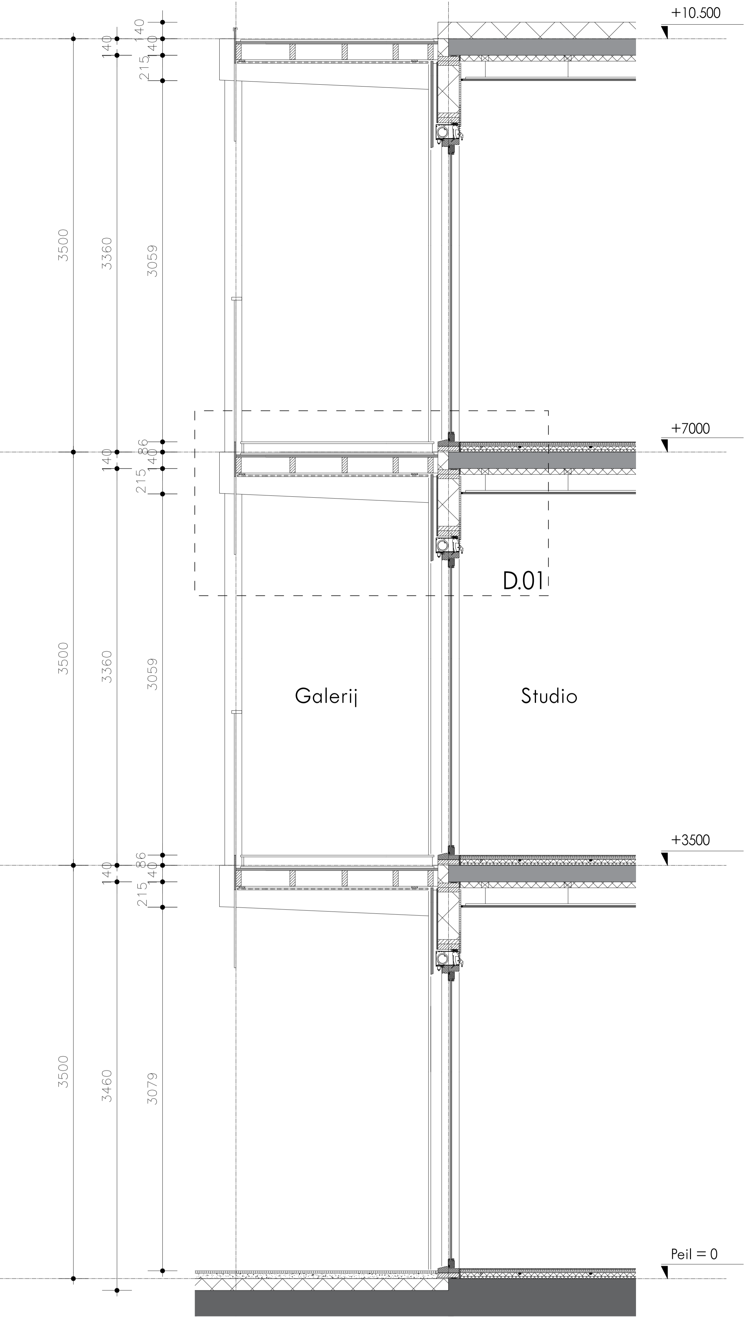
UITWERKING WAND Lengte-, dwars- en horizontale doorsnede wand
