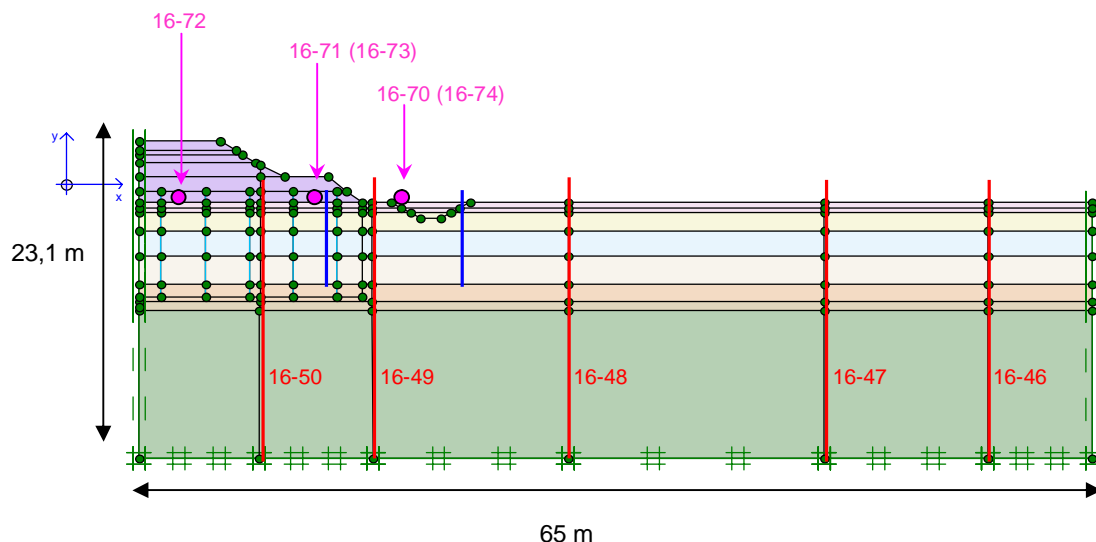
Figuur 7.1 Dwarsdoorsnede Plaxis met locaties meetinstrumenten
