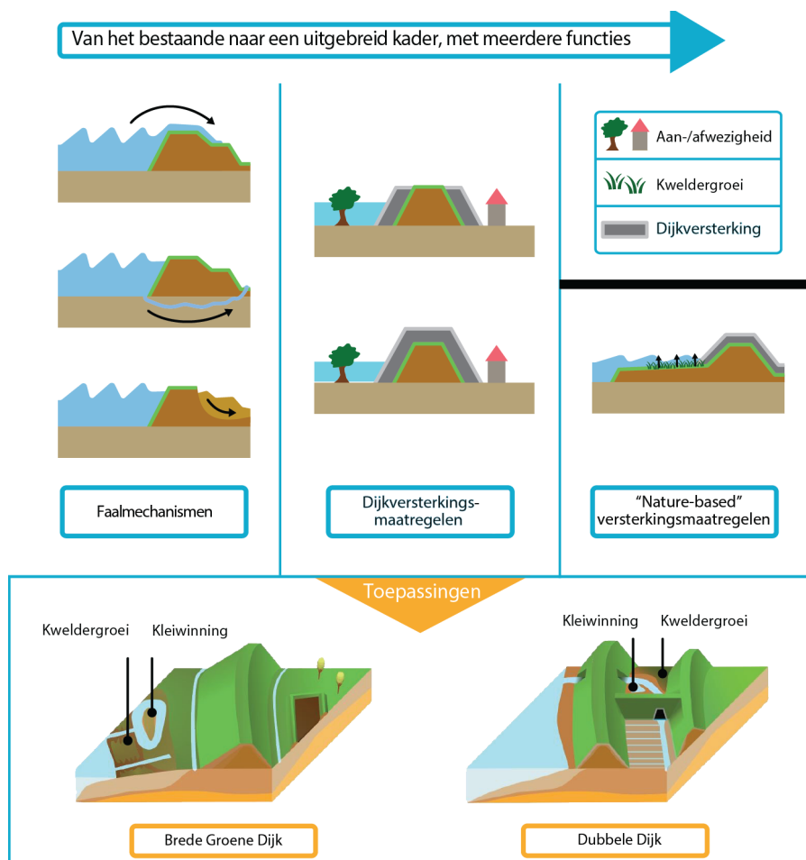
Figuur 3: Onderzoeksc componenten voor het bepalen van een beoordelingskader met medegebruik binnen de nieuwe overstromingsrisicobenadering. Gebaseerd op schema's van Richard Marijnissen.
