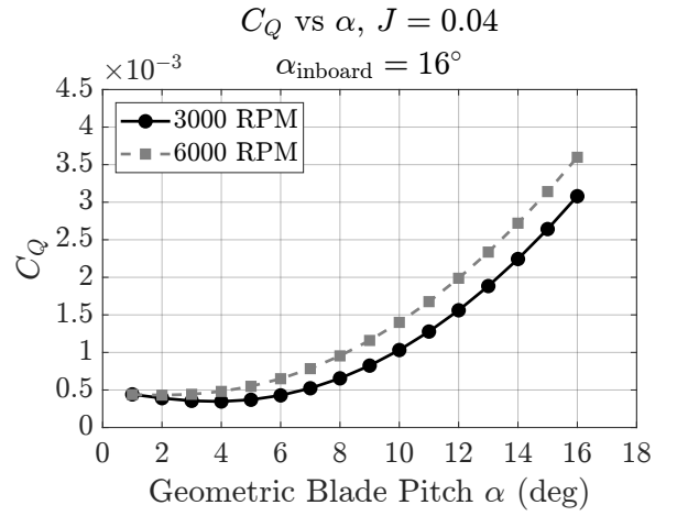
(d) C_Q vs. \alpha at J = 0.04
