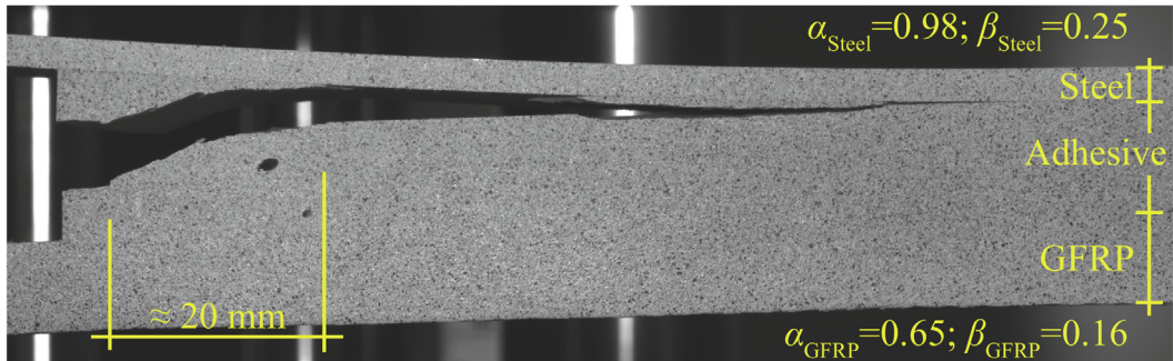
(d) Crack trajectory in steel-GFRP joint - cohesive fracture onset.
