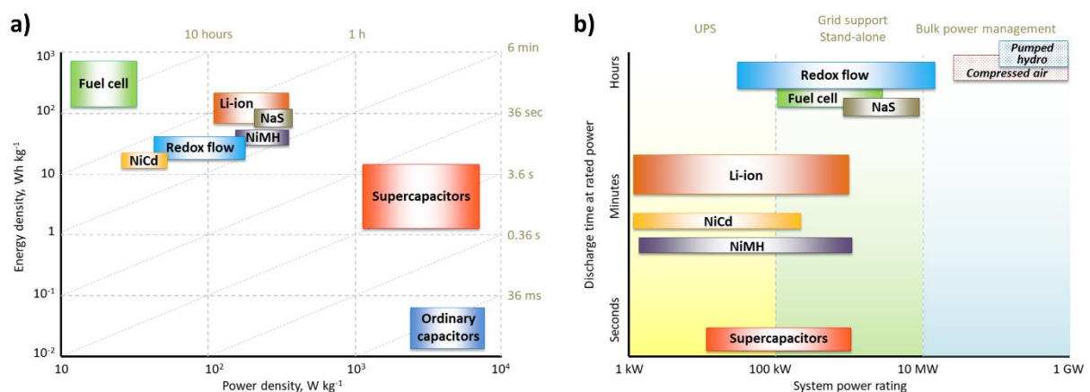
그림 5. 저장 매체에 따른 일률밀도(power density) 및 에너지밀도(energy density)(a)와 방전량 및 방전시간(b) 차트. Ref. [21]와 [22]를 참조하여 작성함.
